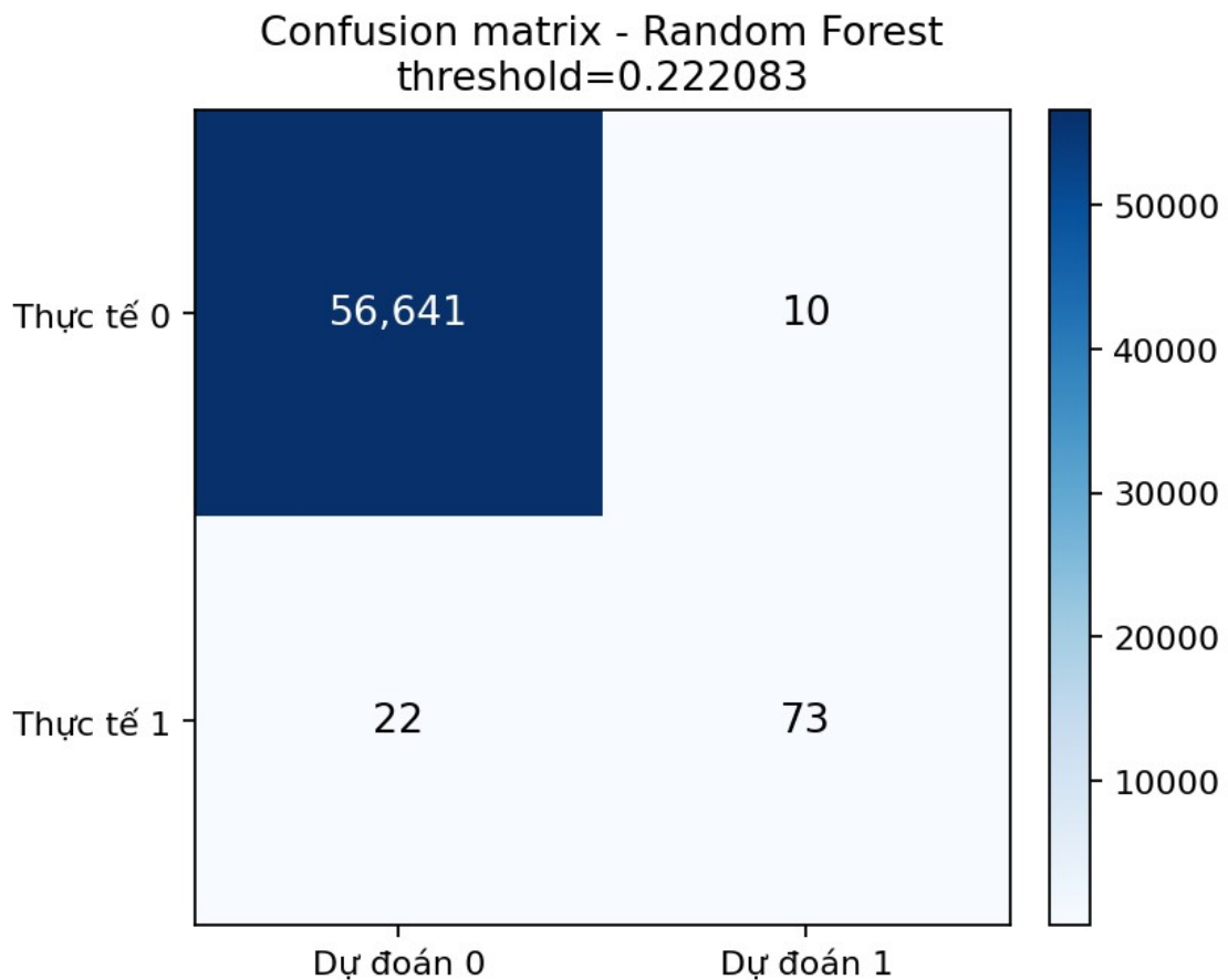
Hình 3.8. Confusion matrix tại threshold đã khóa
