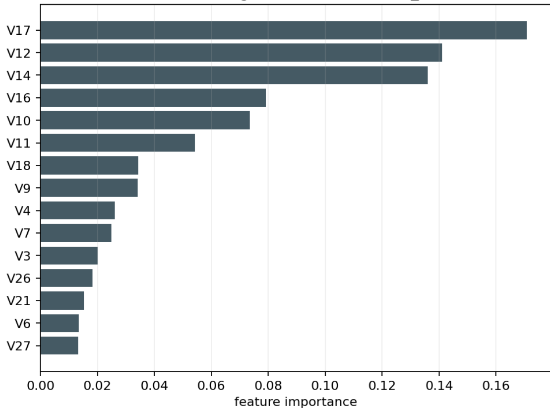
Hình 3.10. Feature importance của Random Forest
