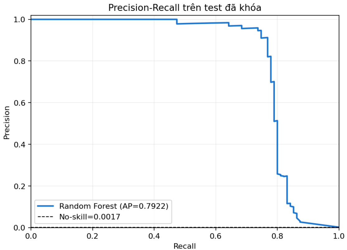
Hình 3.7. Precision-Recall trên test đã khóa
