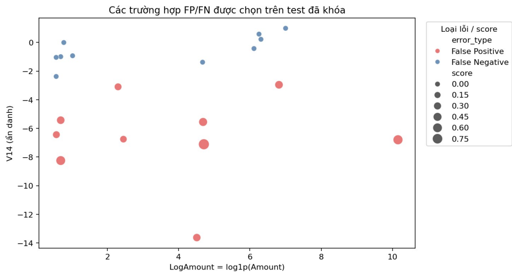
Hình 3.10. Seaborn đa biến trên mẫu FP/FN của test đã khóa
