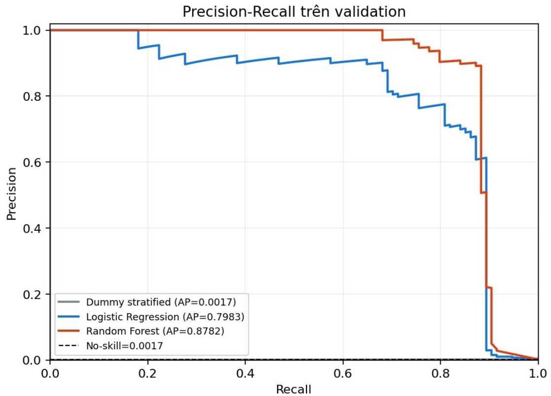
Hình 3.6. Precision Recall trên validation
