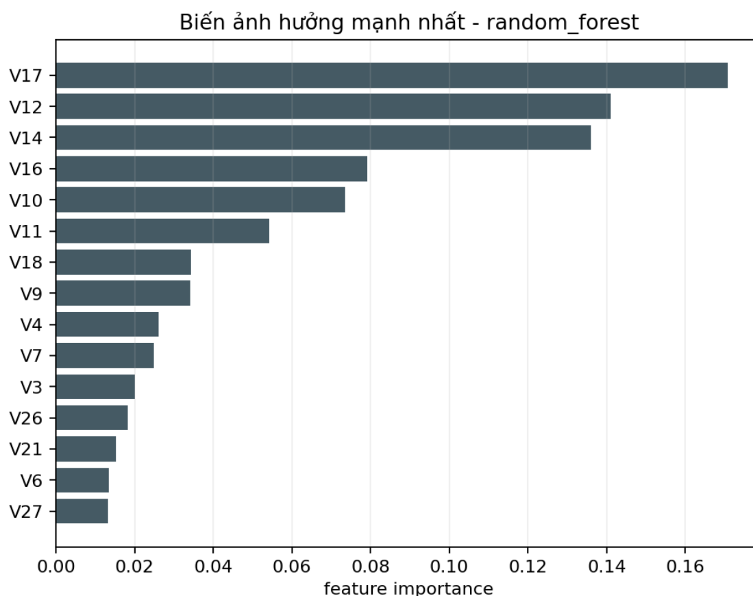
Hình 3.11. Feature importance của Random Forest
