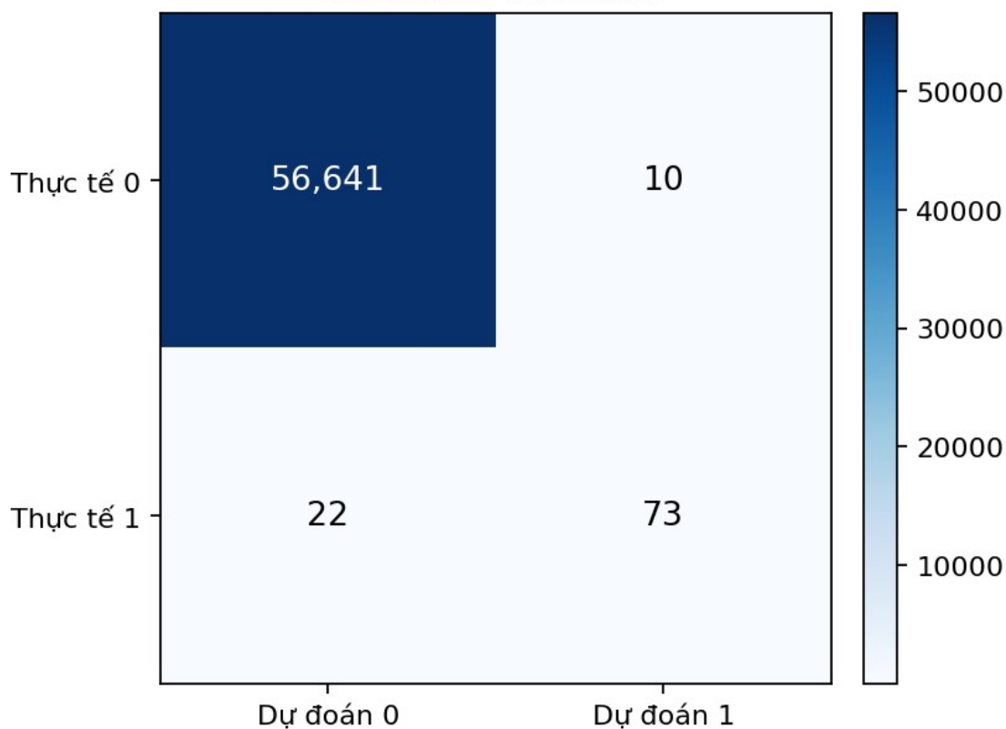
Hình 3.8. Confusion matrix tại threshold đã khóa Confusion matrix - Random Forest threshold=0.222083
