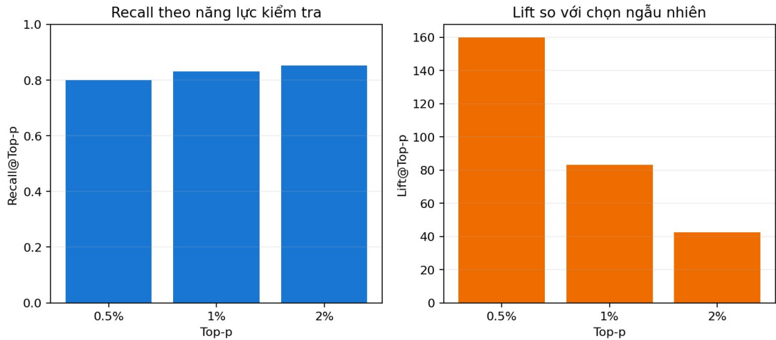
Hình 3.9. Recall và Lift theo Top-p
