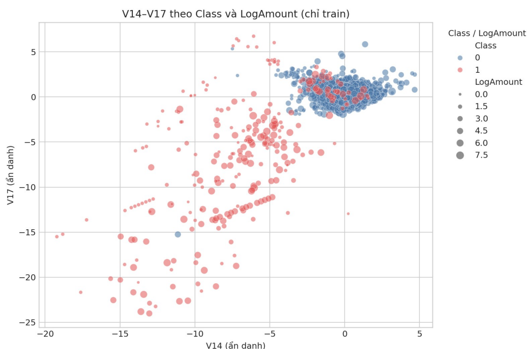
Hình 3.5. Seaborn đa biến trên train
