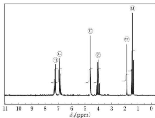
[ ^1H NMR 스펙트럼 (90 MHz, CDCl_3 )]
