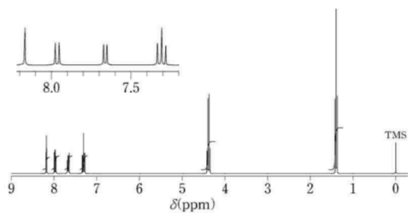
[ ^1H NMR 스펙트럼 (300 MHz, CDCl_3 )]
