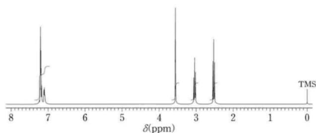
[ C 의 ^1\text{H} NMR 스펙트럼 (300 MHz, \text{CDCl}_3 )]
