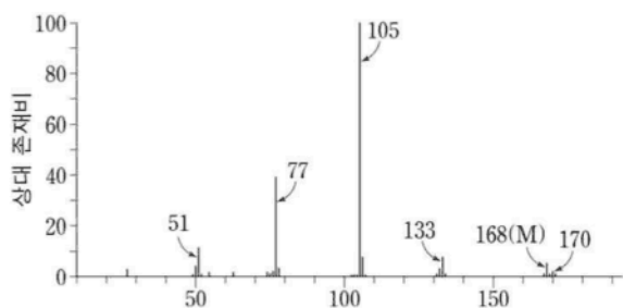
[질량 스펙트럼]
