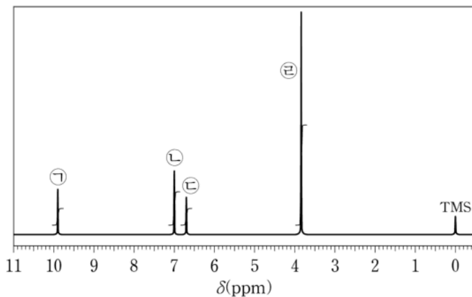
[ ^1H NMR 스펙트럼 (90MHz, CDCl_3 )]
