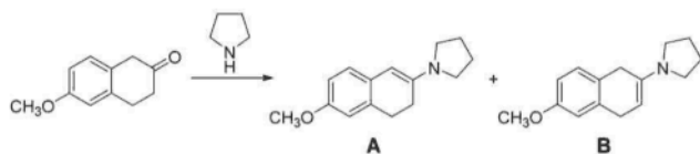
[반응 1]
