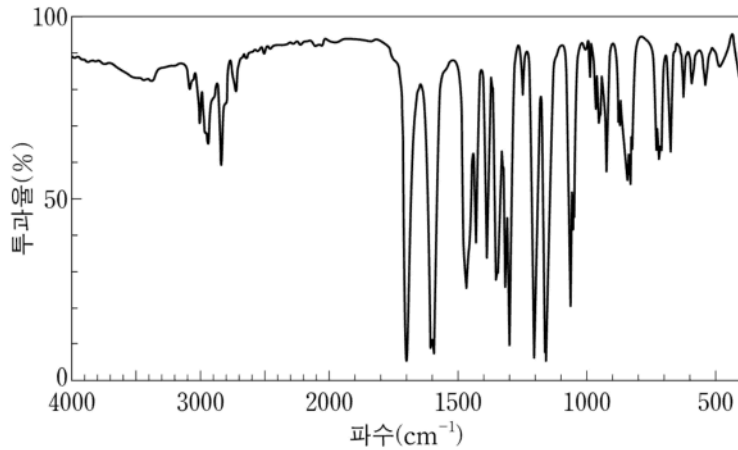
[IR 스펙트럼]
