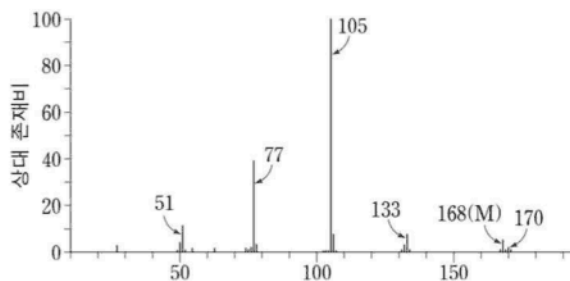
[질량 스펙트럼]
