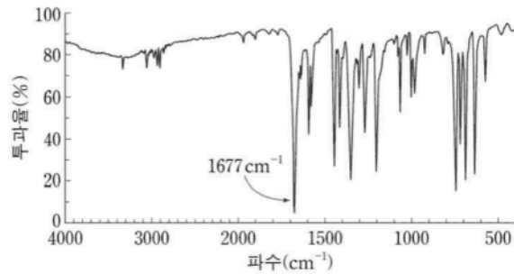
[IR 스펙트럼]
