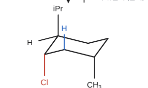
C의 모두 축 형태: anti H는 CH 2 쪽(파랑) 1곳뿐 (iPr 탄소의 H는 적도) → 2-menthene만, 느림
