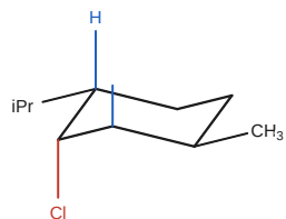
A의 가장 안정한 의자형 iPr·CH 3 적도, Cl 축(아래) → 바로 E 2 가능 Cl 양옆 C의 축 H(위, 파랑) 2개가 Cl과 anti
