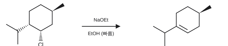
B: 3-menthene (주생성물, Zaitsev)
