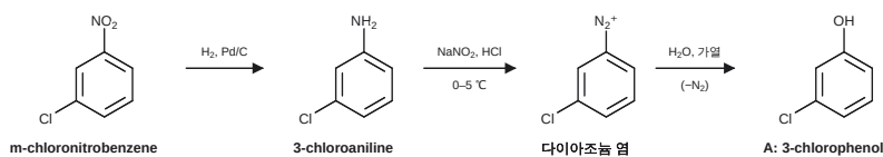
[반응 1] 다이아조늄 경유 페놀 합성
