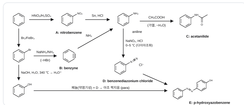
벤젠 유도체 합성 경로도의 A~E
