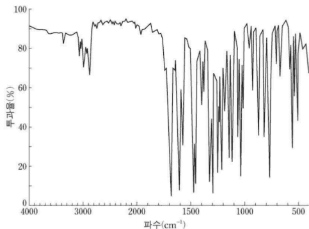
[IR 스펙트럼]
