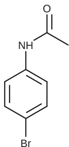
B: 4-bromoacetanilide (p-)
