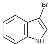
C: 3-bromoindole (C 8 H 6 NBr)
