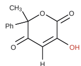
토토머 ① (C 3 엔올)
