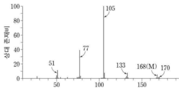
[질량 스펙트럼]
