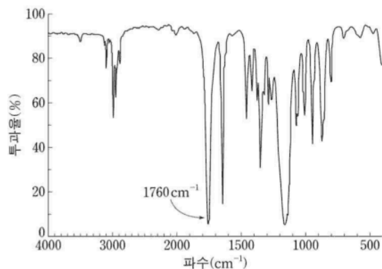
[IR 스펙트럼]
