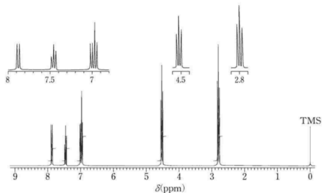
[ ^1H NMR 스펙트럼(300 MHz, CDCl_3 )]
