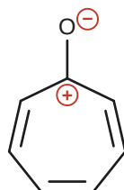
A의 방향족 공명 구조 (6 \pi , tropylium)
