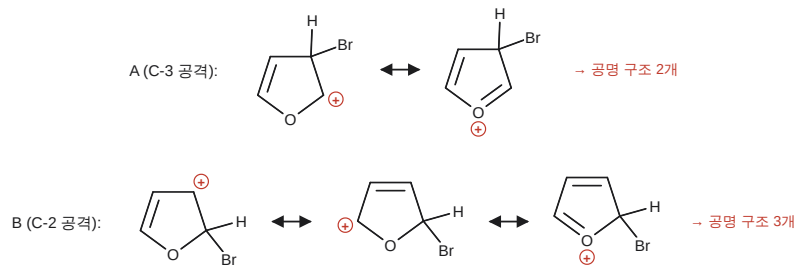
중간체 A, B의 공명 구조
