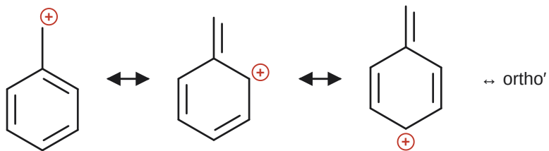
벤질 양이온의 공명
