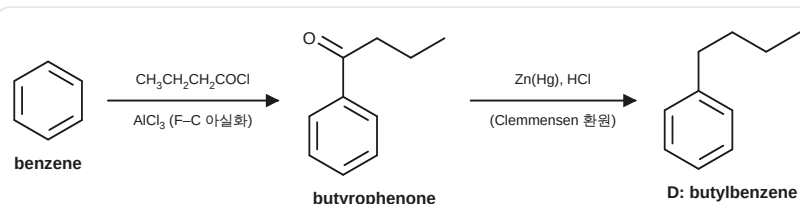
D의 2단계 합성
