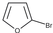
D: 2-bromofuran (주)
