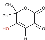
토토머 ② (C 5 엔올)
