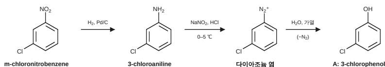
[반응 1] 다이아조늄 경유 페놀 합성
