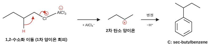
[반응 3] 1,2-수소화 이동과 C 생성
