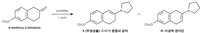
[반응 1] 엔아민의 위치 이성질체
