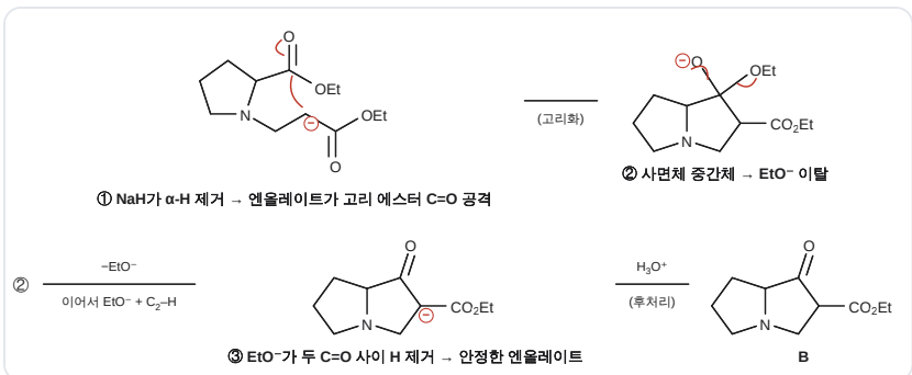
A → B Dieckmann 메커니즘
