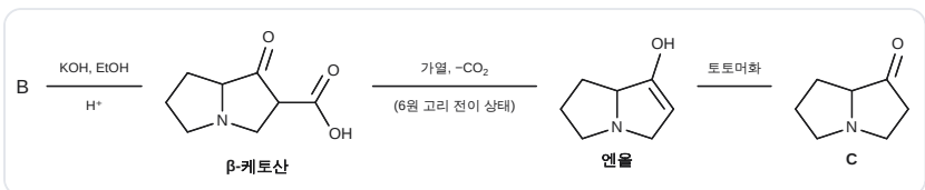
B → C: 비누화·탈카복실화
