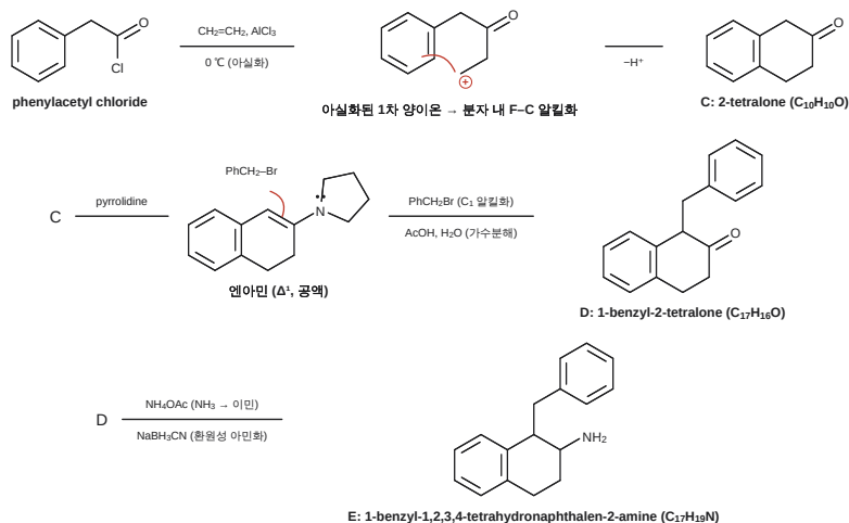
[반응 2] C → D → E
