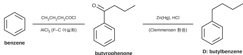
D의 2단계 합성
