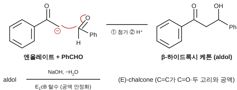
Claisen-Schmidt 축합 핵심 단계
