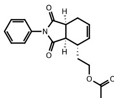
B' (exo)
