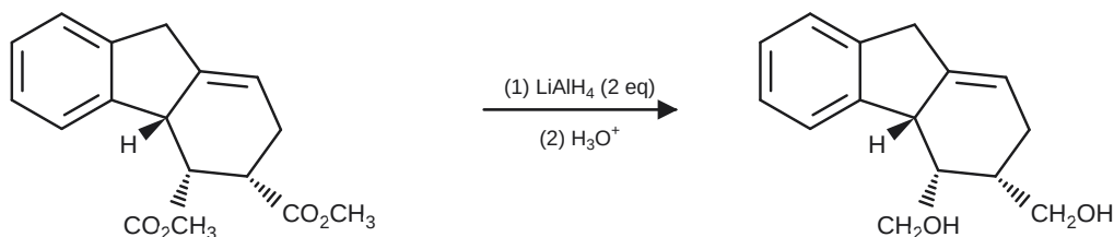
DA 부가물 (두 에스터 cis)
