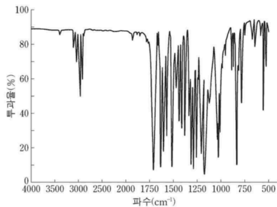
[IR 스펙트럼]
