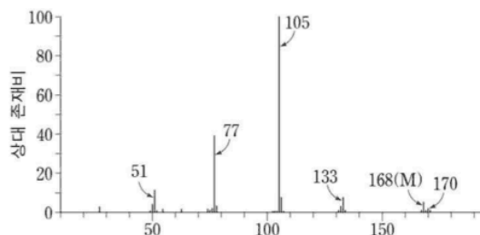
[질량 스펙트럼]
