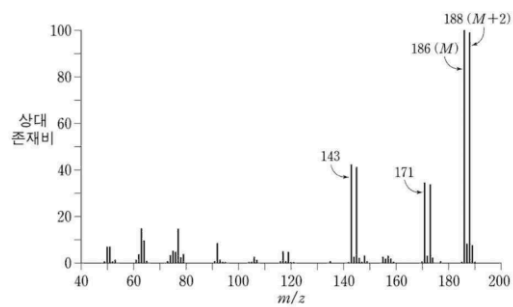
질량 스펙트럼
