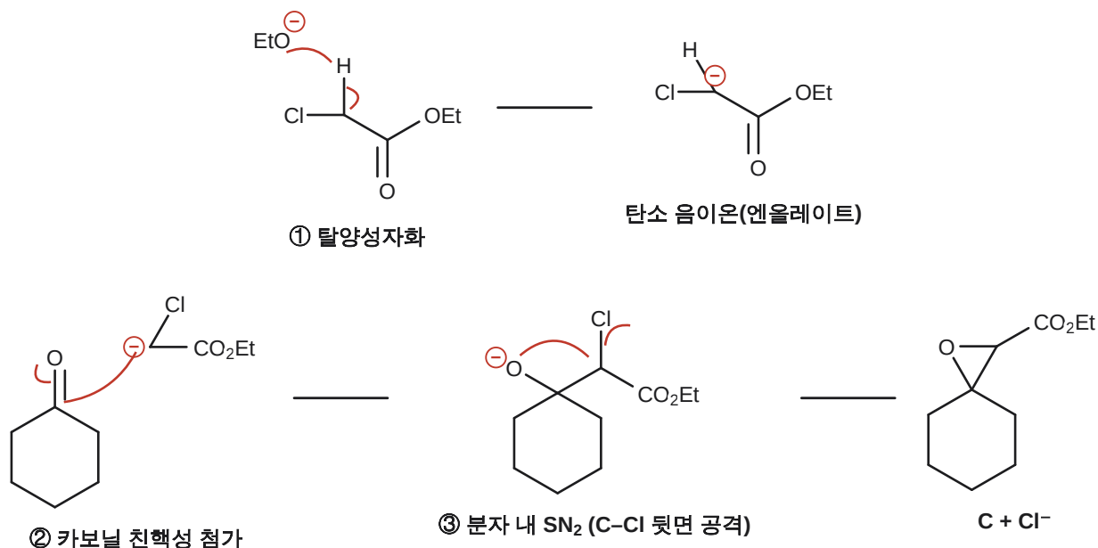
C 생성 메커니즘 (굵은 화살표)
