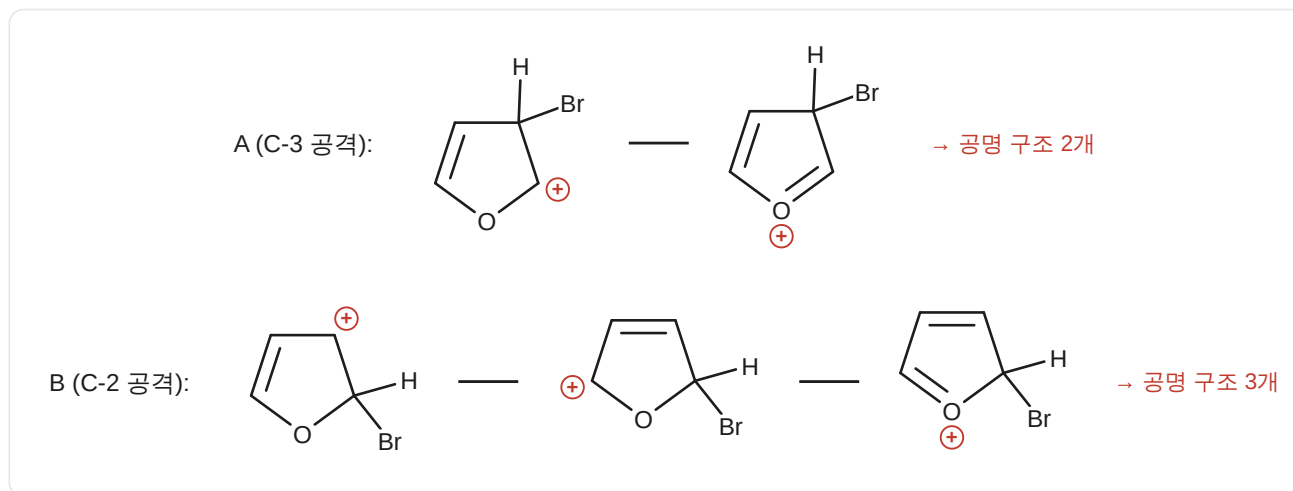
중간체 A, B의 공명 구조
