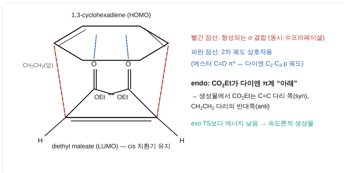
endo 전이 상태 (2차 궤도 상호작용)
