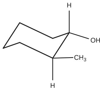
E: trans-2-methylcyclohexanol — OH·CH 3 모두 적도
