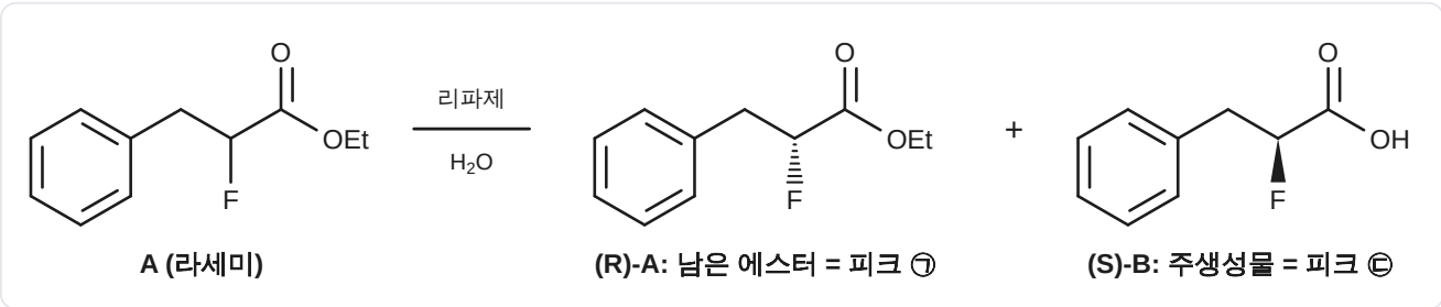
리파제에 의한 속도론적 광학 분할
