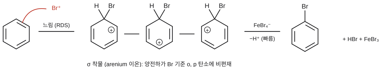
1-2: \text{FeBr}_3 촉매 브로민화 — \sigma 착물(arenium) 공명과 탈양성자화
