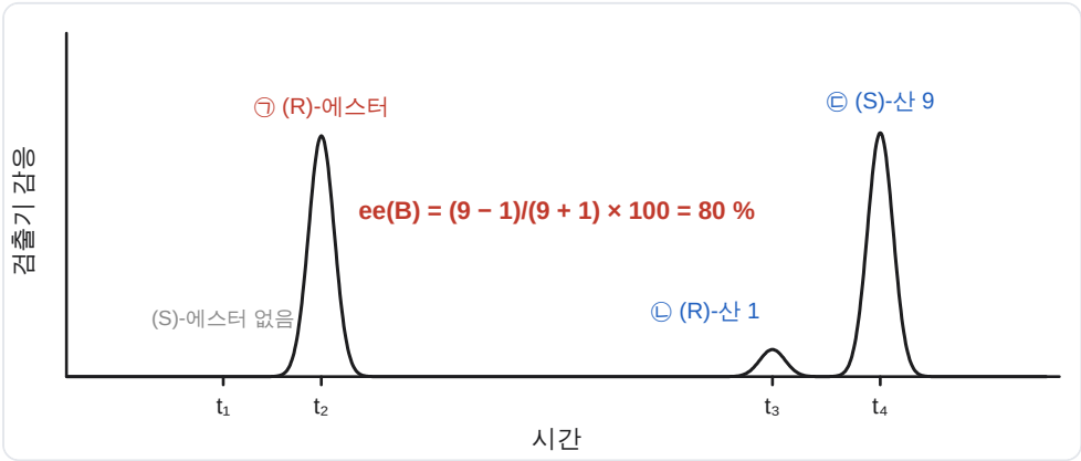
반응 후 혼합물의 카이랄 크로마토그램 해석
