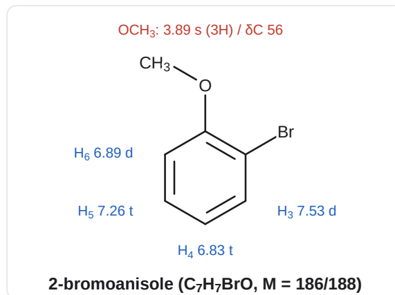
2-bromoanisole의 ^1\text{H} 귀속
