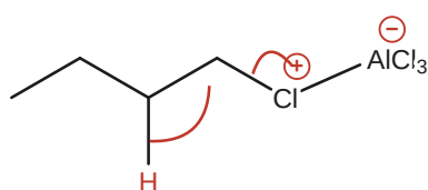
1,2-수소화 이동 (1차 양이온 회피)
