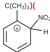
ortho 공격 σ 착물
