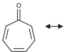
A: tropone
