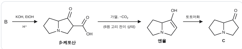
B → C: 비누화·탈카복실화
