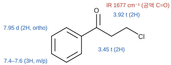
A: 3-chloro-1-phenylpropan-1-one ( \text{C}_9\text{H}_9\text{ClO} )
