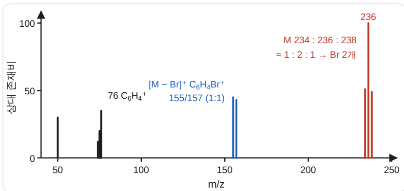
질량 스펙트럼 해석 (개형)
