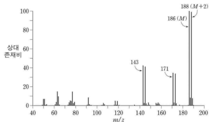
질량 스펙트럼
