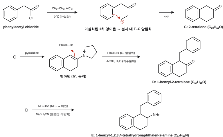
[반응 2] C \rightarrow D \rightarrow E
