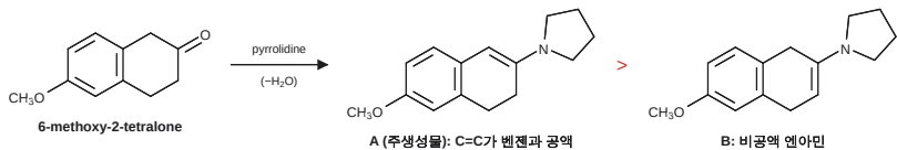
[반응 1] 엔아민의 위치 이성질체
