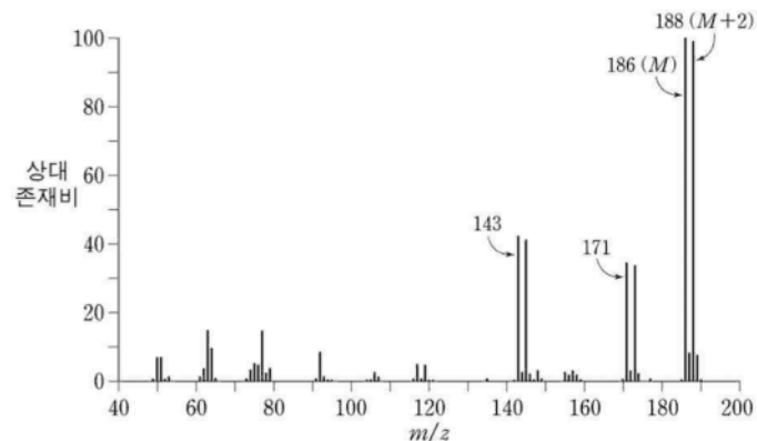
질량 스펙트럼
