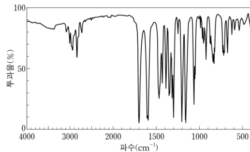
[IR 스펙트럼]
