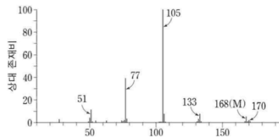
[질량 스펙트럼]
