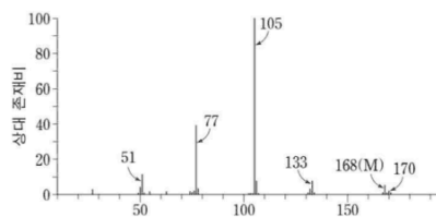
[질량 스펙트럼]
