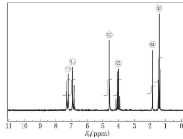
[ ^1H NMR 스펙트럼 (90MHz, CDCl_3 )]
