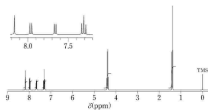
[ ^1H NMR 스펙트럼 (300 MHz, CDCl_3 )]
