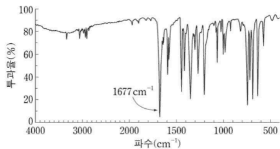
[IR 스펙트럼]
