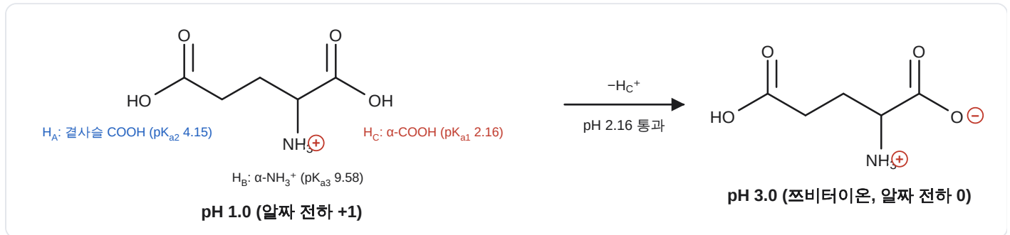
pH 1.0과 pH 3.0의 우세 구조
