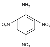
2,4,6-trinitroaniline pK a H ≈ -9.4 (최소)
