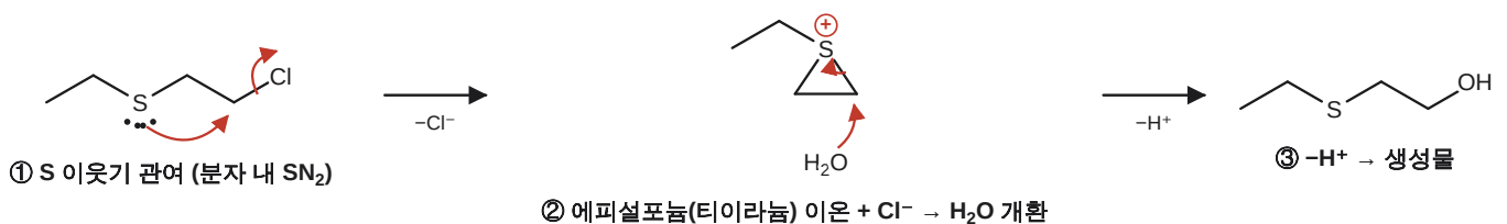
B의 이웃기 관여 메커니즘
