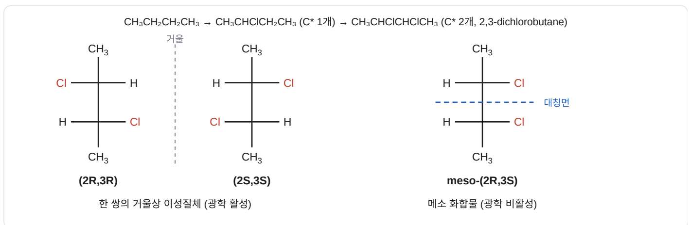
2,3-dichlorobutane의 입체 이성질체 3개 (Fischer 투영)
