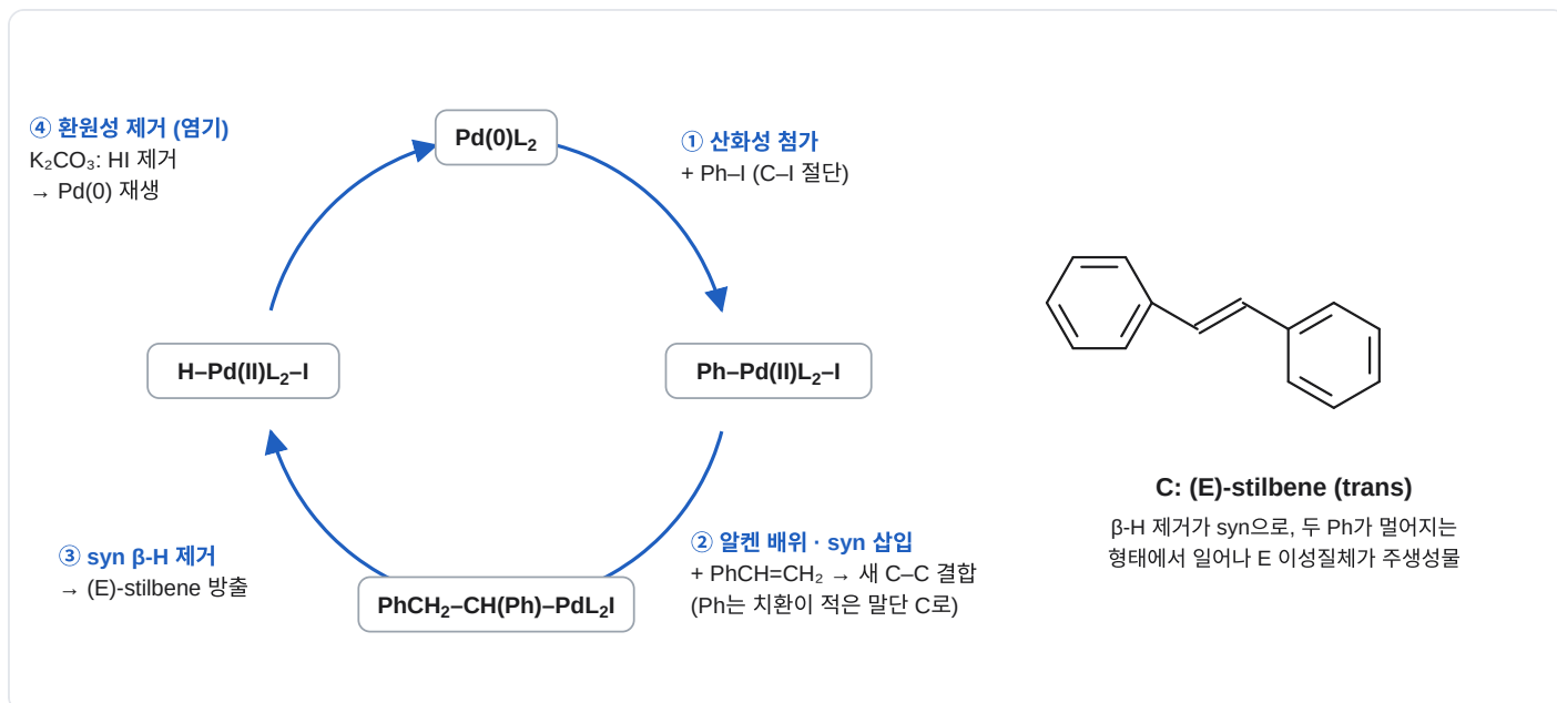
반응 III: Heck 반응의 Pd 촉매 순환과 생성물 C
