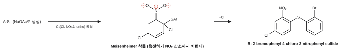
[반응 2] SNAr (첨가-제거)
