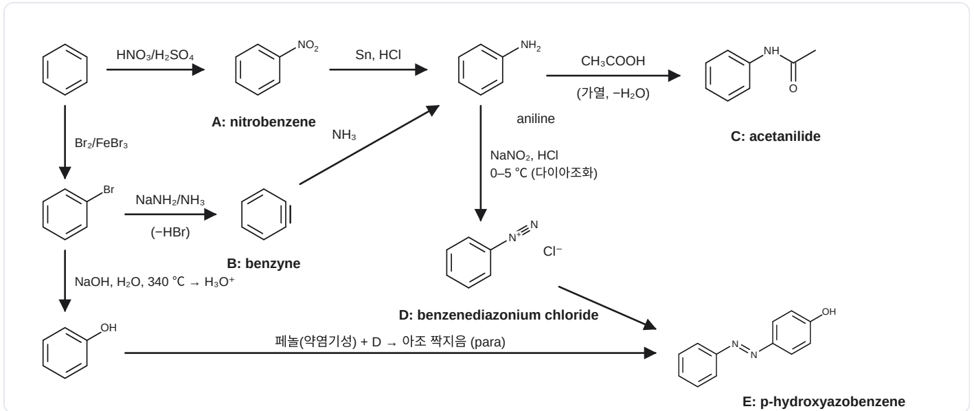
벤젠 유도체 합성 경로도의 A~E
