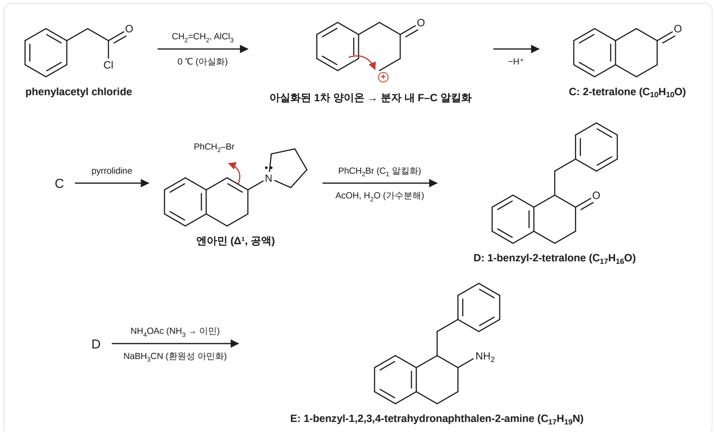
[반응 2] C → D → E
