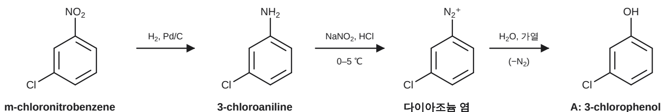
[반응 1] 다이아조늄 경우 페놀 합성
