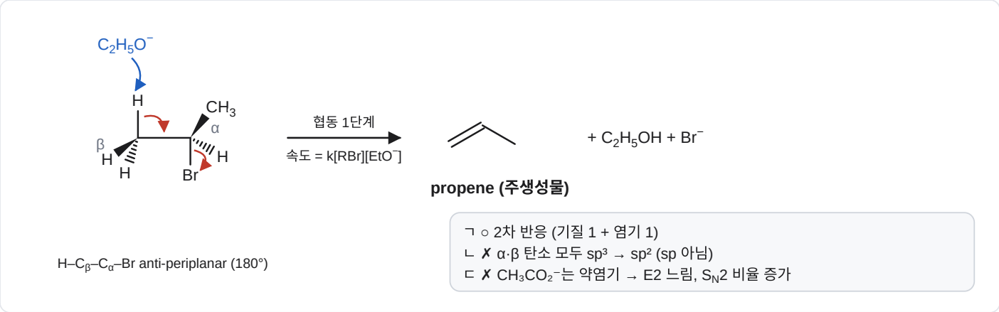
2-bromopropane의 E2: anti-periplanar 배치와 굵은 화살표, 보기 판정
