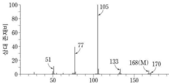
[질량 스펙트럼]
