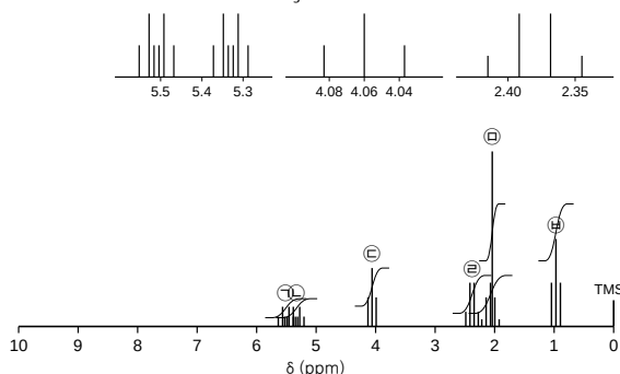
[ ^1H NMR 스펙트럼(300 MHz, CDCl_3 )]
