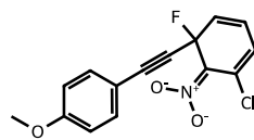
중간체(Meisenheimer 착물)
