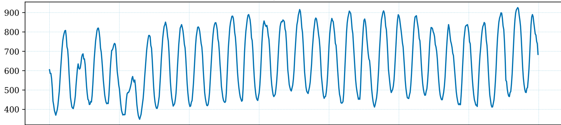
Trend
