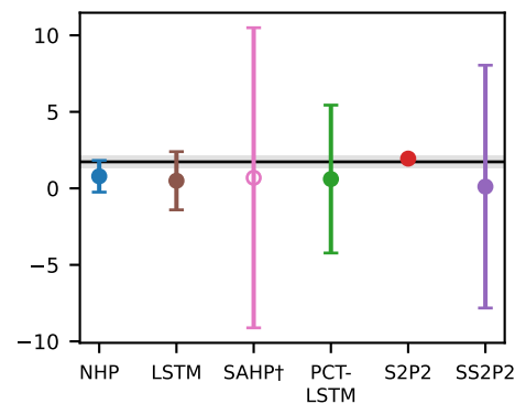
F3 return skewness
