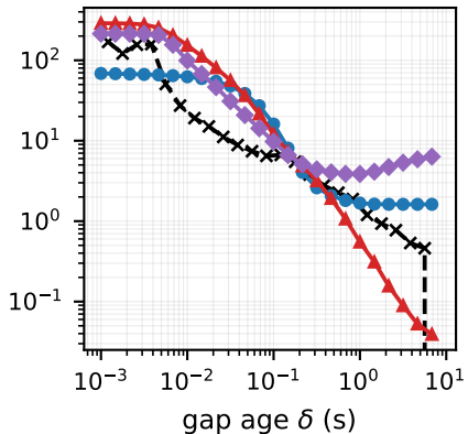
SOL
