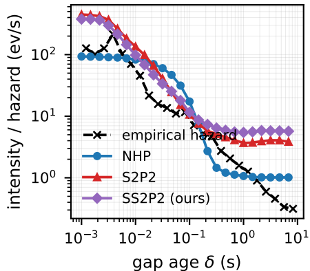
BTC
