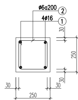
MẶT CẮT 1-1
