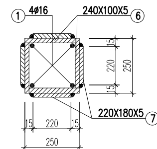
MẶT CẮT 2-2
