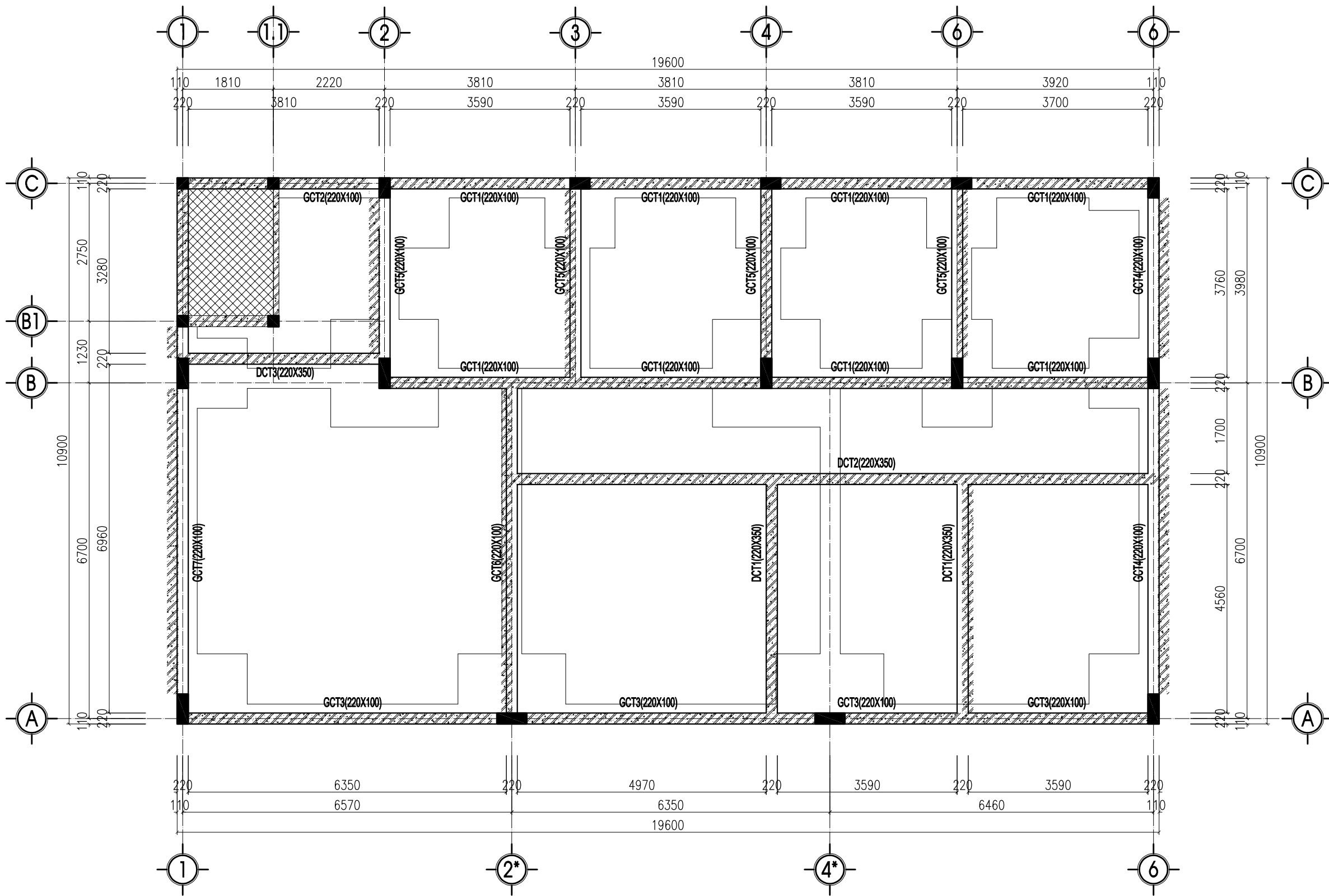
MẶT BẰNG GIẢNG CHÂN TƯỜNG + DẦM CHÂN TƯỜNG
