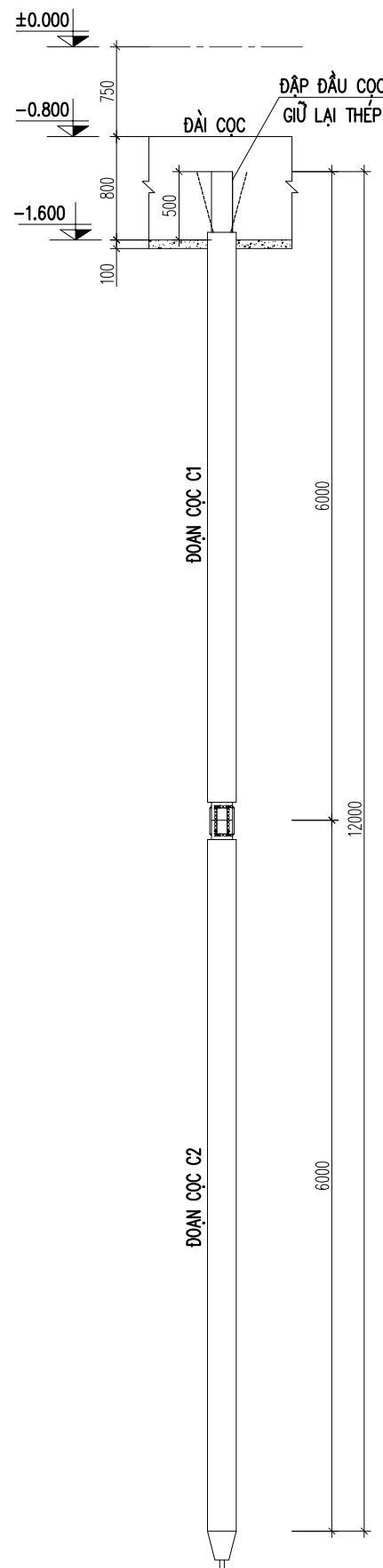
SƠ ĐỒ CỌC ĐẠI TRÀ
