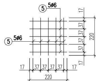
LƯỚI S1
