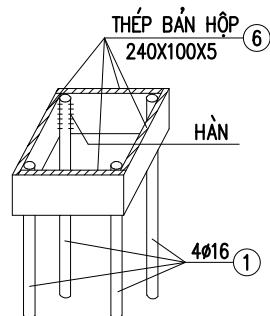
CHI TIẾT HÀN THÉP BÀN ĐẦU CỌC
