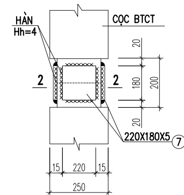
CHI TIẾT NỐI CỌC
