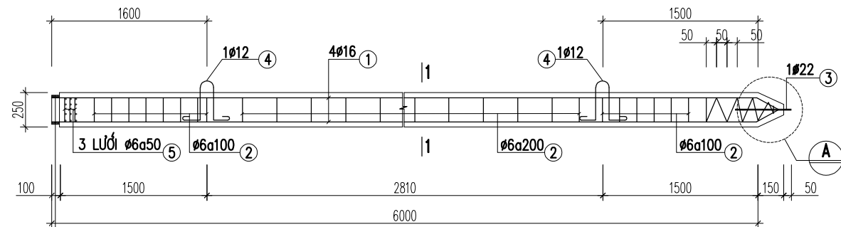
ĐOẠN CỌC MŨI C2 (1 ĐOẠN)
