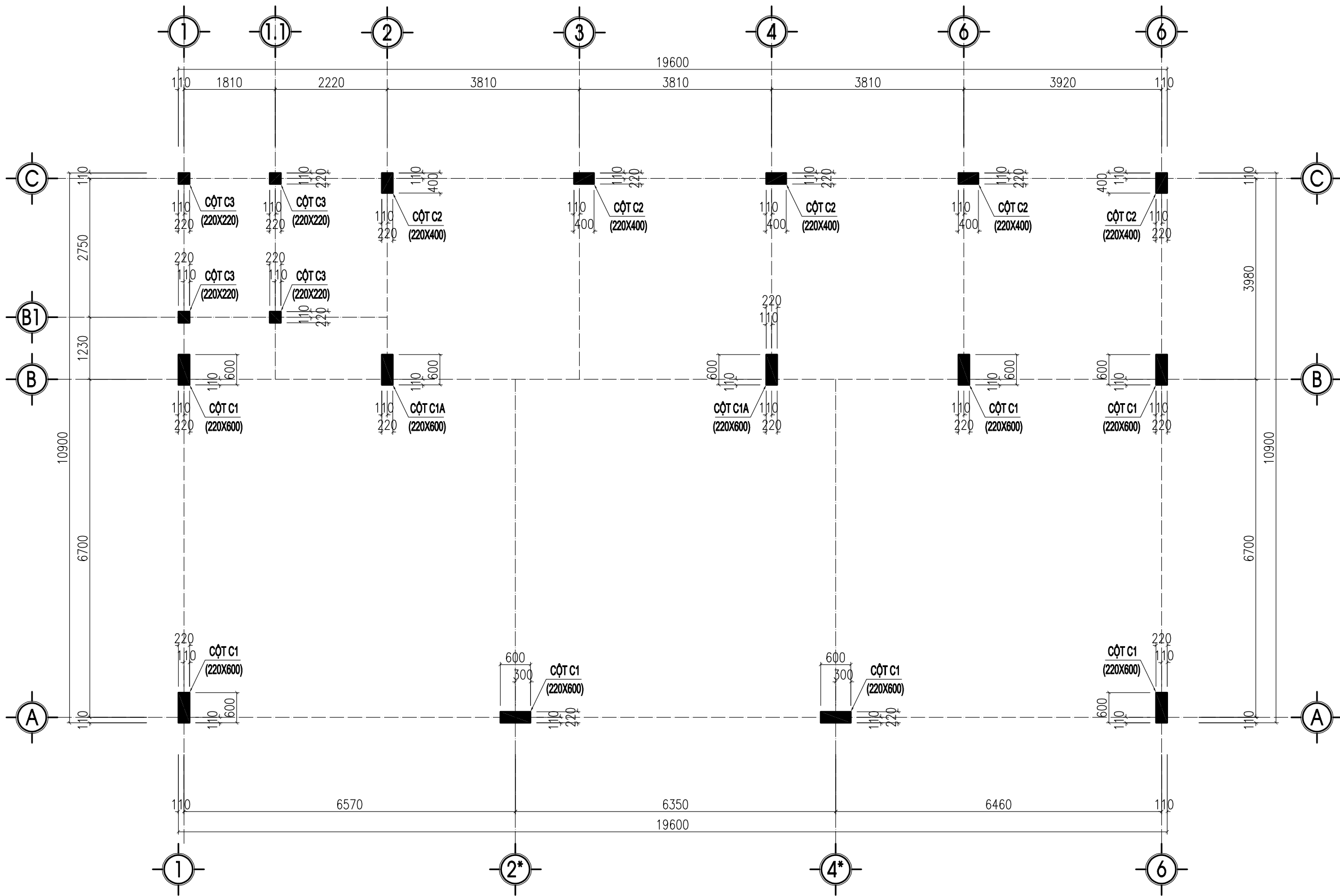
MẶT BẰNG ĐỊNH VỊ CỘT TẦNG 1
