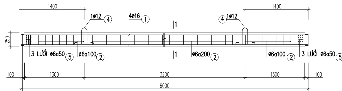
ĐOẠN CỌC THÂN C1 (1 ĐOẠN)
