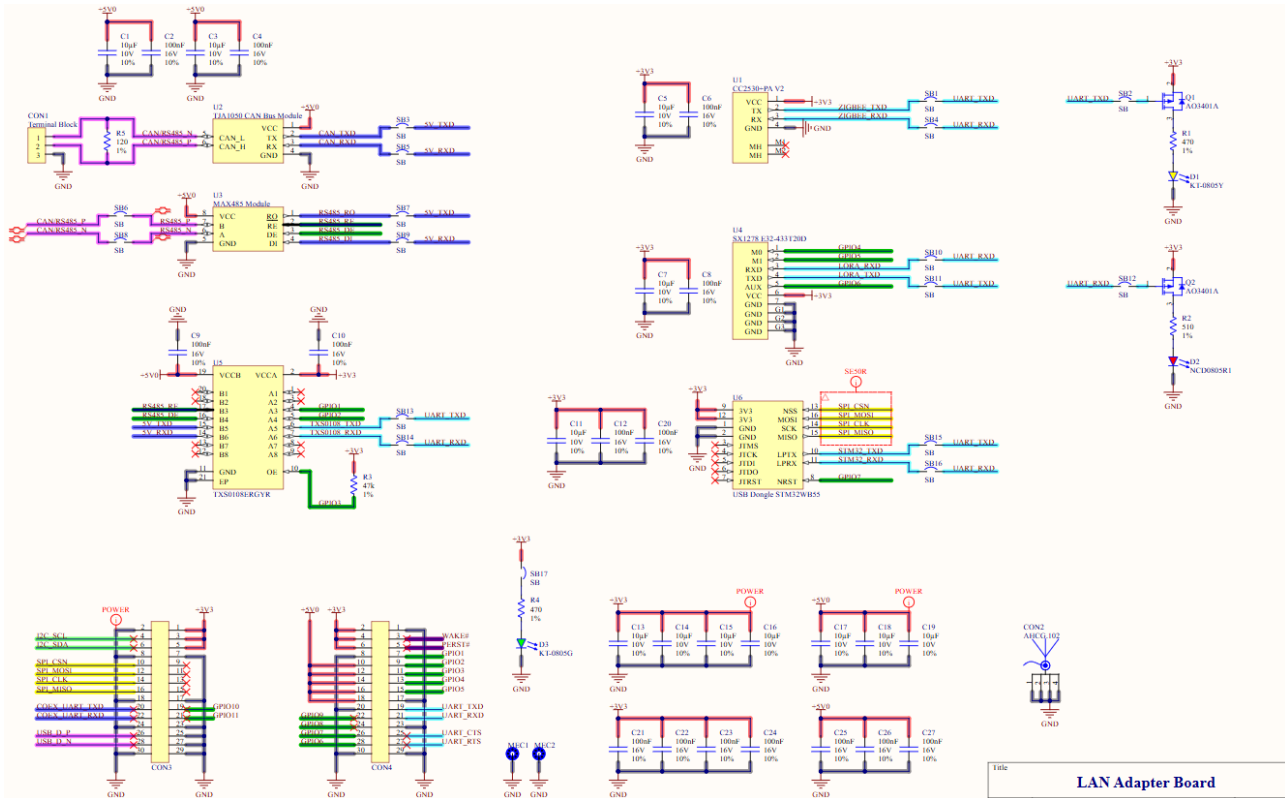
Hình 4.19: Sơ đồ nguyên lý mạch LAN Adapter
