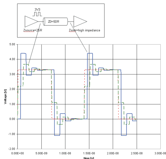
Hình 3.4: Minh hoạ hiện tượng ringing do không khớp trở kháng
