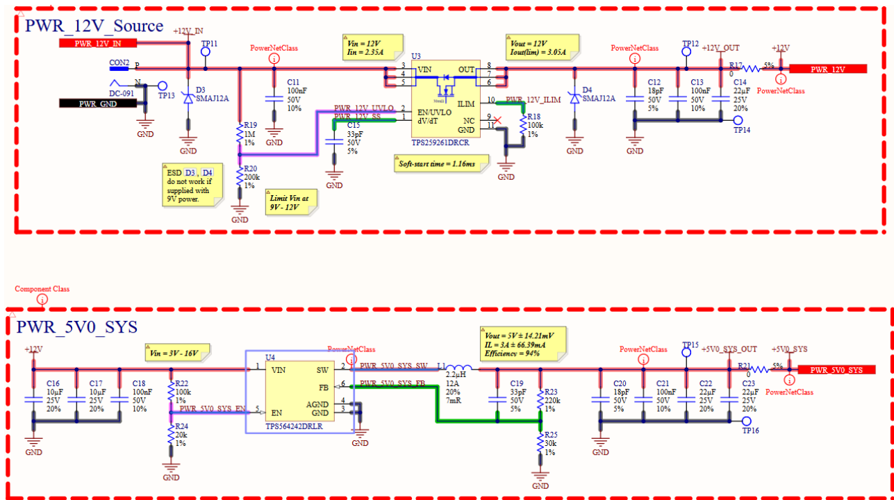
Hình 4.8: Sơ đồ nguyên lý mạch nguồn 1
