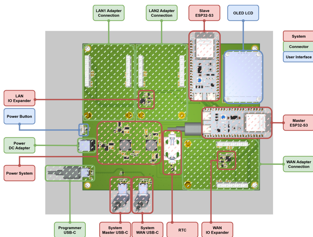
Hình 6.1: Assembly Diagram.
