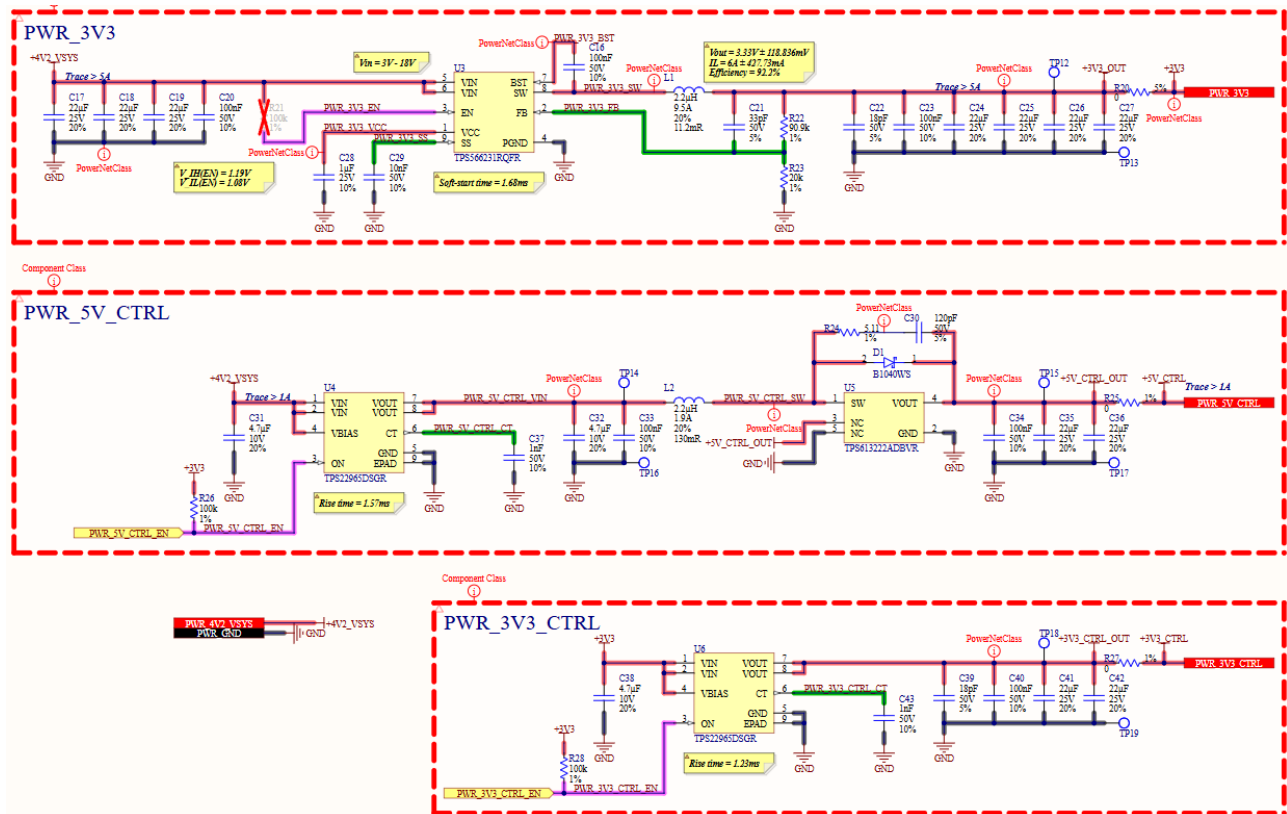
Hình 4.16: Sơ đồ nguyên lý mạch nguồn DC-DC
