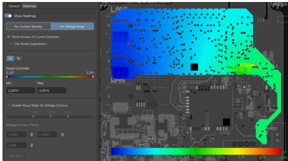
Hình 4.70: Biểu đồ phân bố điện áp trên nguồn +3V3_CTRL.
