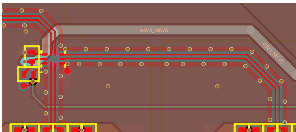
Hình 4.10: Kỹ thuật bọc mass và stitching via dọc theo đường tín hiệu USB tốc độ cao.
