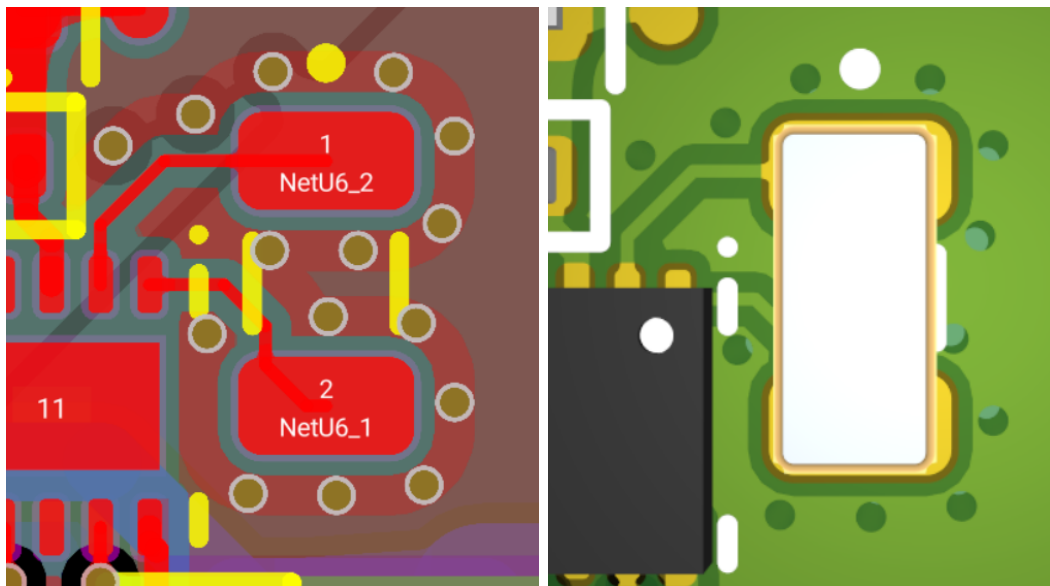
Hình 4.11: Phủ GND Shielding và stitching via xung quanh thạch anh.
