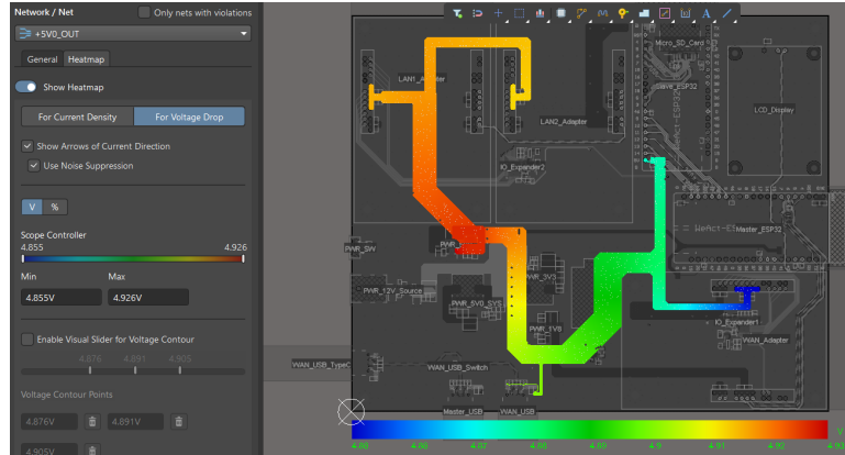
Hình 4.31: Biểu đồ phân bố điện áp (Voltage Drop Heatmap) trên nguồn +5V0.
