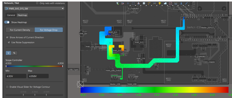
Hình 4.30: Biểu đồ phân bố điện áp (Voltage Drop Heatmap) trên nguồn +5V0_SYS.
