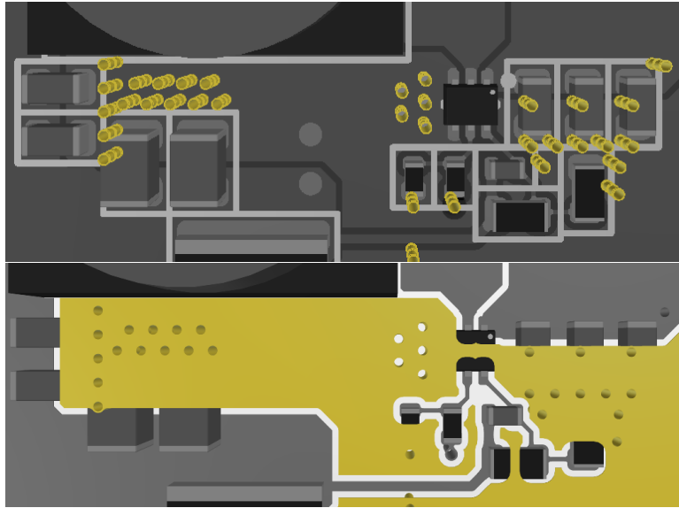
Hình 4.19: Tản nhiệt trong nguồn xung +5V0_SYS.
