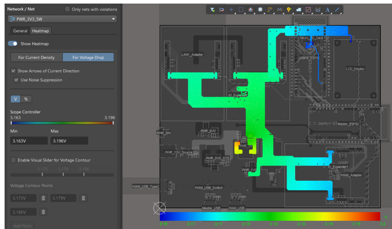
Hình 4.32: Biểu đồ phân bố điện áp (Voltage Drop Heatmap) trên nguồn +3V3.
