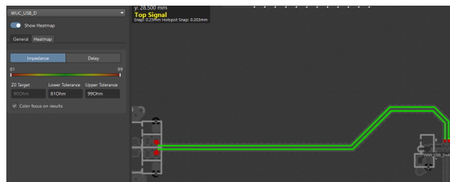
Hình 4.26: Biểu đồ phân bố trở kháng (Impedance Heatmap) đường vi sai.
