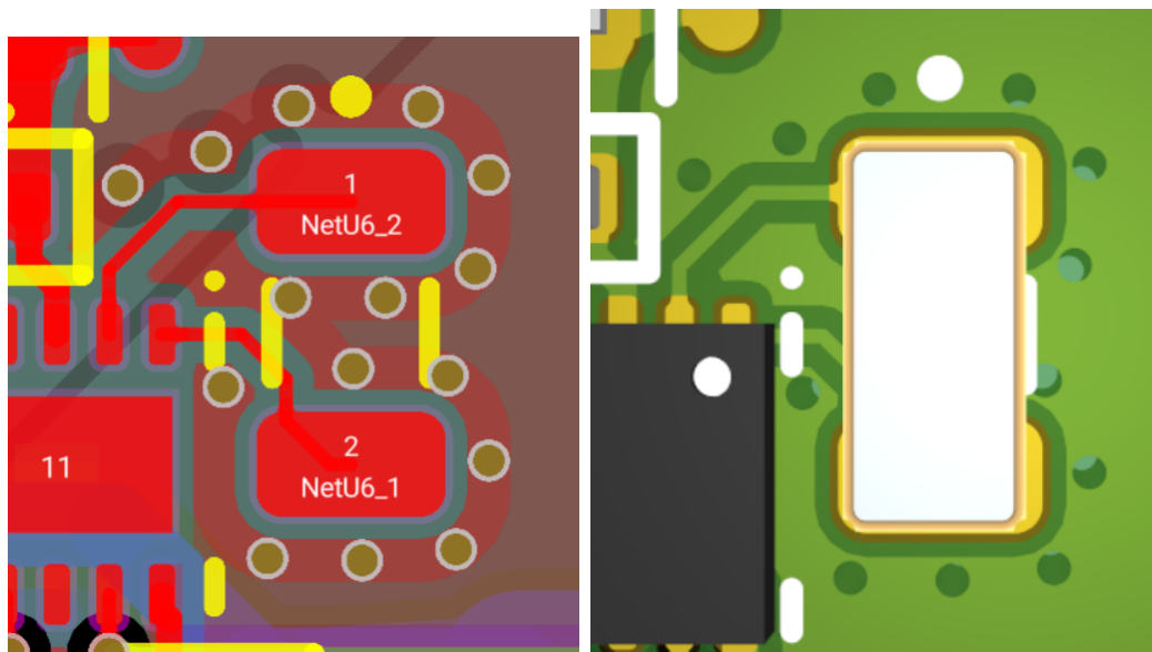
Hình 4.13: Kỹ thuật tạo vòng bảo vệ (Guard Ring) và via stitching xung quanh khối thạch anh để cô lập nhiễu.
