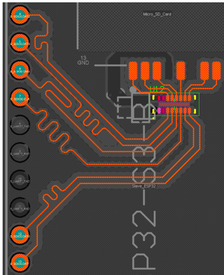
Hình 4.22: Định tuyến SDIO giữa ESP32-S3 Slave với Micro SD Card.
