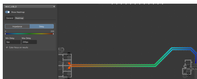
Hình 4.27: Biểu đồ phân bố độ trễ lan truyền (Propagation Delay) đường vi sai.
