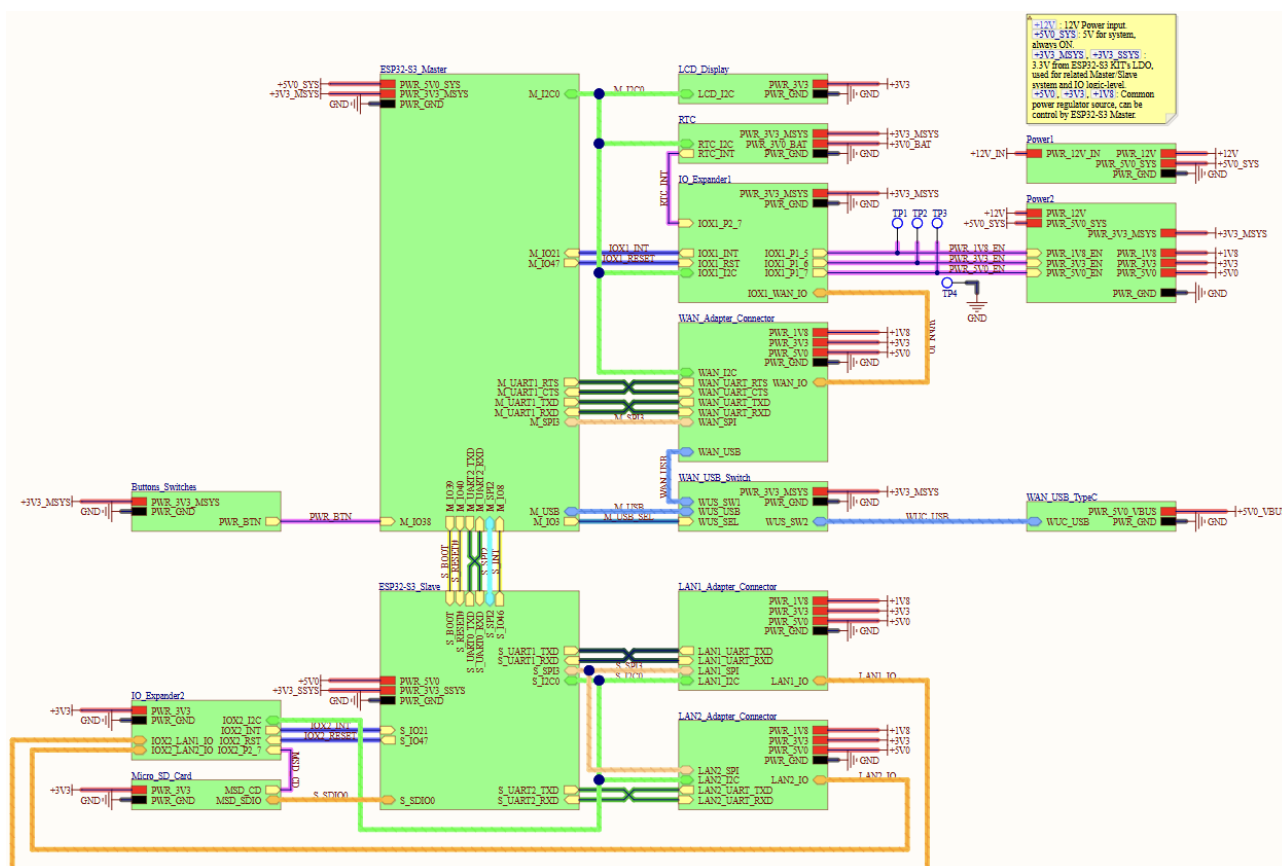
Hình 4.9: Sơ đồ nguyên lý hệ thống
