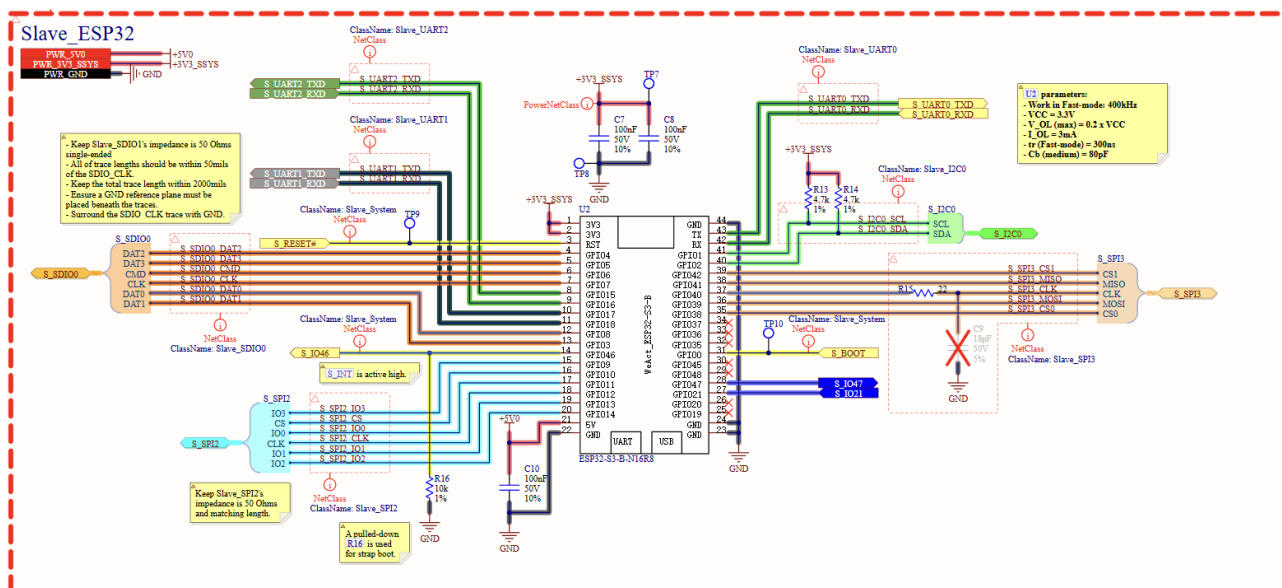
Hình 4.10: Sơ đồ nguyên lý ESP32 Slave
