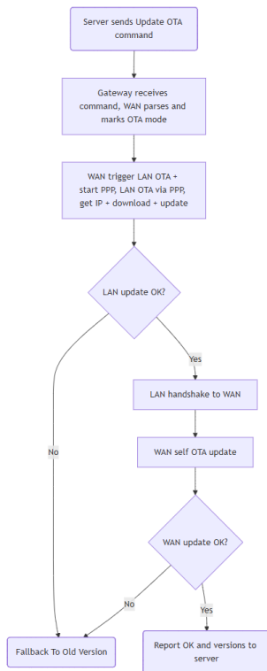
Hình 4.52: Lưu đồ giải thuật FOTA cho Dual-MCU Gateway
