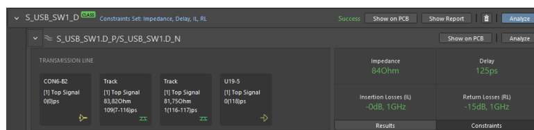
Hình 4.58: Bảng tổng hợp thông số mô phỏng đường vi sai.
