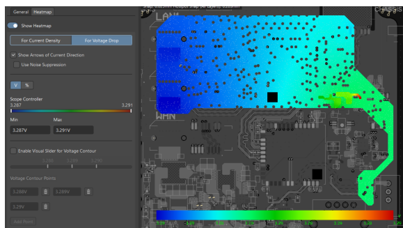
Hình 4.73: Biểu đồ phân bố điện áp trên nguồn +3V3_CTRL.
