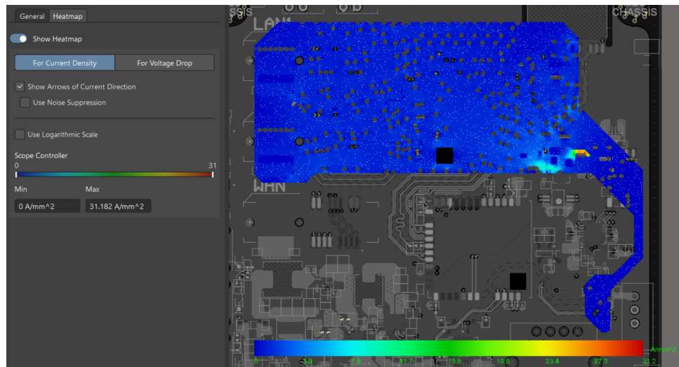
Hình 4.72: Biểu đồ phân bố mật độ dòng điện của nguồn +3V3_CTRL.
