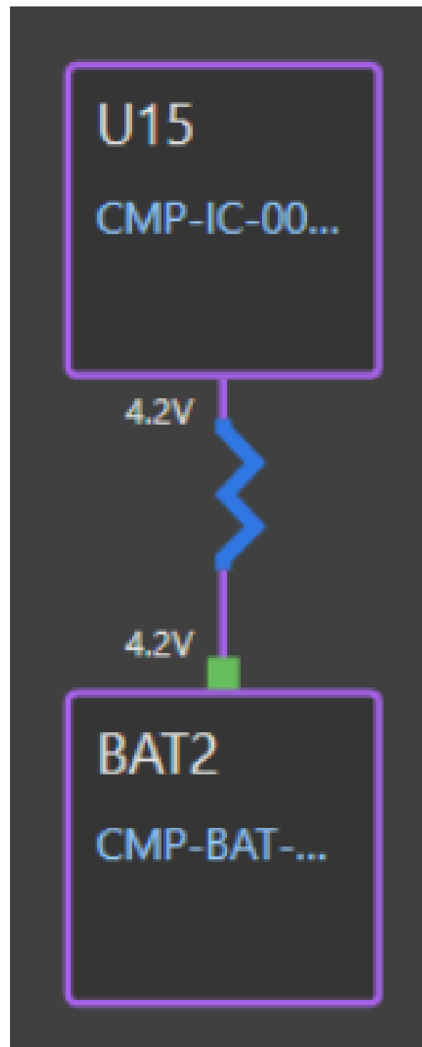
Hình 4.71: Cây phân phối nguồn +3V7_VBAT.
