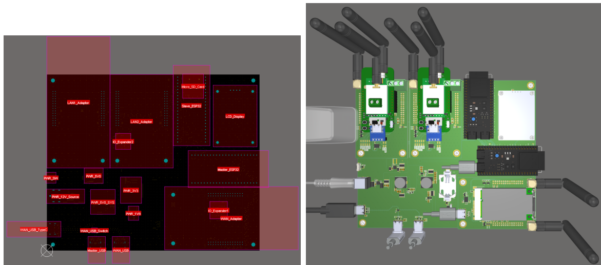
Hình 4.37: Sơ đồ quy hoạch phân vùng chức năng trên PCB (Floor-planning)
