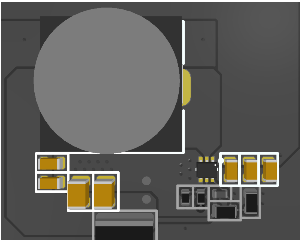
Hình 4.41: Vị trí các tụ điện trong nguồn xung +5V0_SYS.
