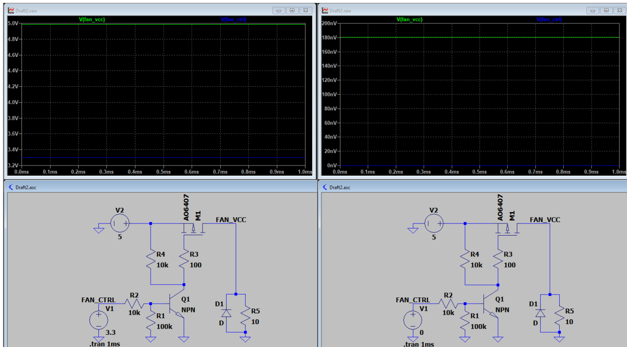
Hình 4.29: Thực hiện mô phỏng mạch điều khiển quat DC trên LTspice
