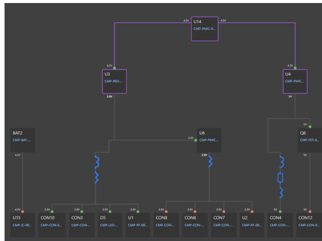
Hình 4.62: Cấu trúc mạng phân phối nguồn.
