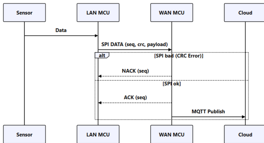
Hình 4.3: Sequence diagram: luồng xử lý dữ liệu end-to-end uplink
