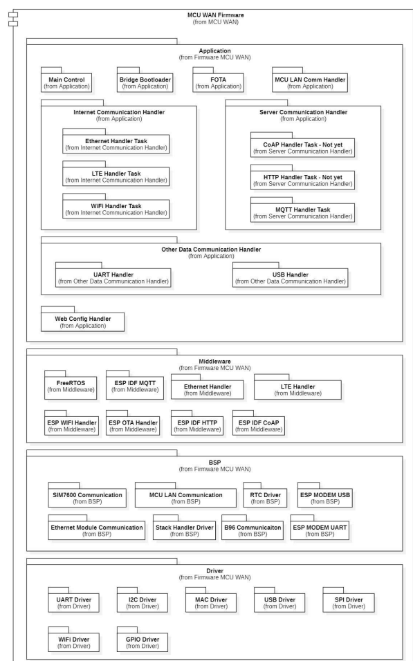
Hình 4.50: MCU WAN Firmware
