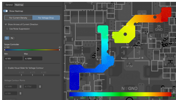
Hình 4.77: Biểu đồ phân bố điện áp trên nguồn +3V7_VBAT.
