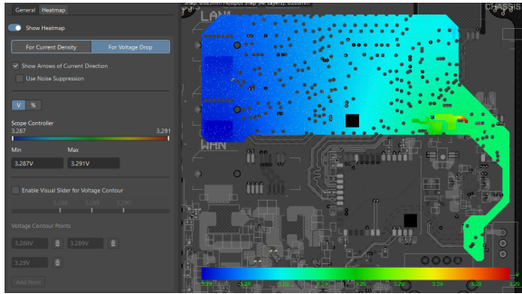
Hình 4.74: Biểu đồ phân bố điện áp trên nguồn +3V3_CTRL.
