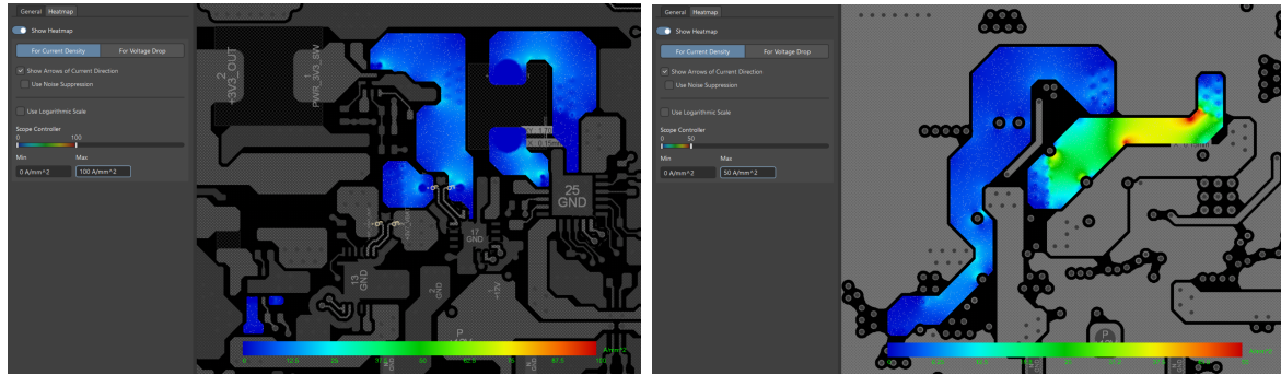
Hình 4.64: Biểu đồ phân bố mật độ dòng điện của nguồn +4V2_VSYS.
