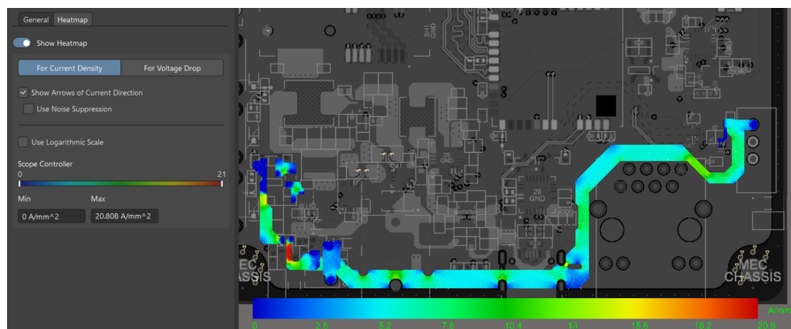
Hình 4.67: Biểu đồ phân bố mật độ dòng điện của nguồn +5V0_CTRL.
