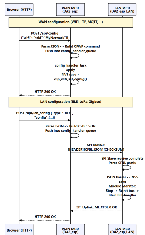
Hình 4.7: Sequence diagram: cập nhật cấu hình từ Web Config Portal
