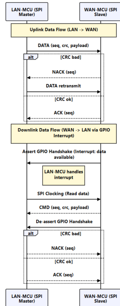
Hình 4.5: Sequence diagram: giao tiếp LAN-MCU ↔ WAN-MCU qua SPI
