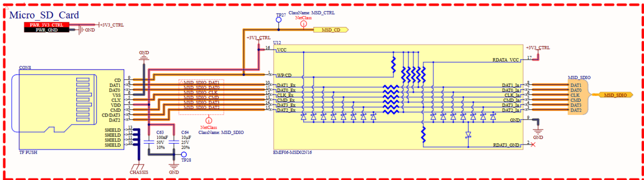
Hình 4.24: Sơ đồ nguyên lý mạch Micro SD Card
