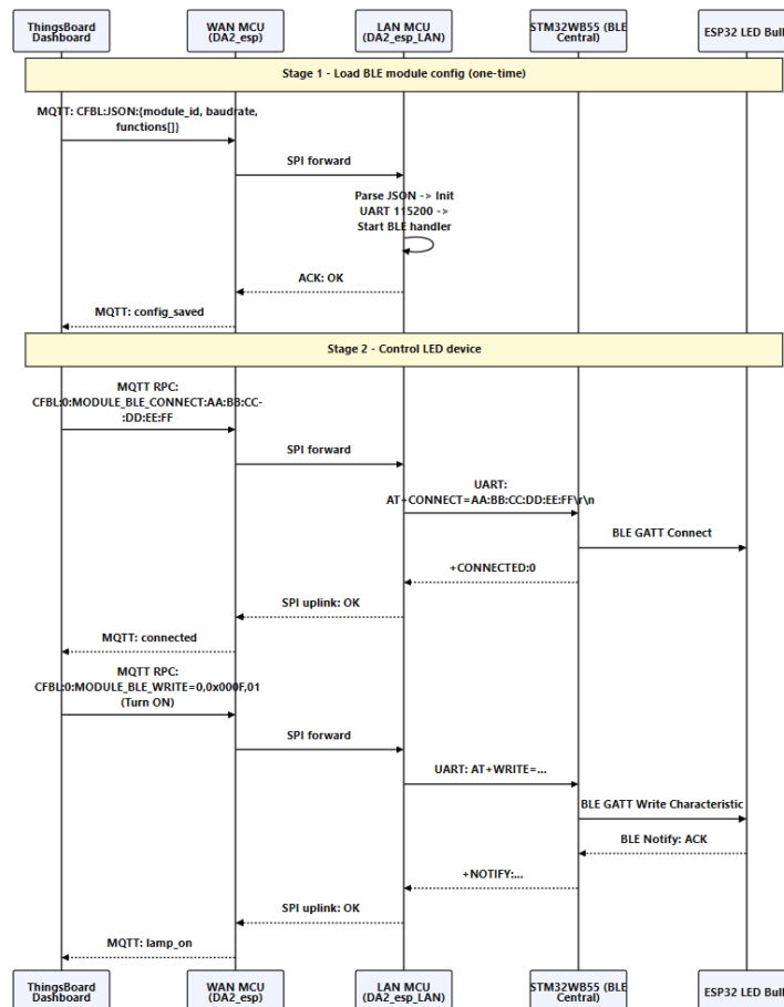
Hình 4.55: Luồng điều khiển end-to-end từ ThingsBoard đến bóng đèn ESP32 qua GW DA2
