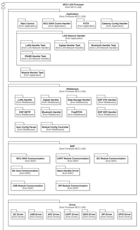
Hình 4.49: MCU LAN Firmware
