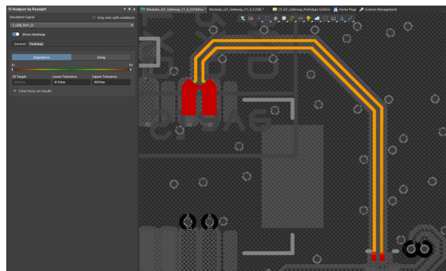
Hình 4.59: Biểu đồ phân bố trở kháng (Impedance Heatmap) đường vi sai.
