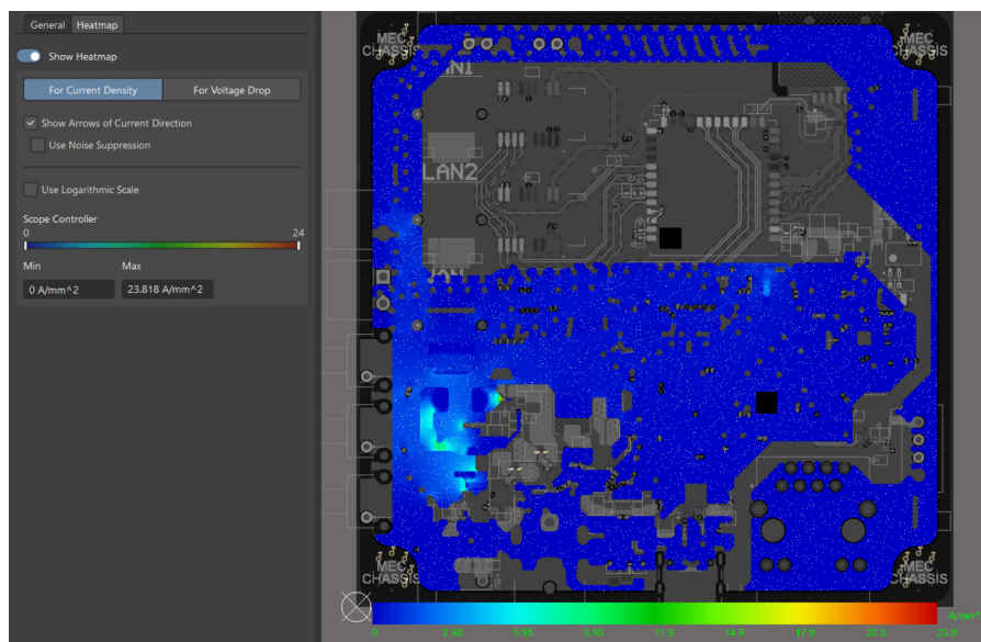
Hình 4.70: Biểu đồ phân bố mật độ dòng điện của nguồn +3V3.
