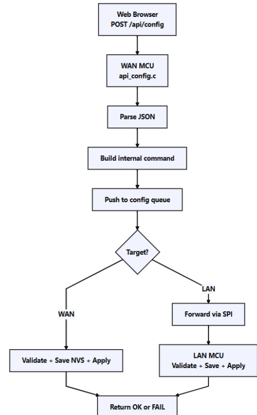
Hình 4.52: Lưu đồ giải thuật Config qua Web Config Portal
