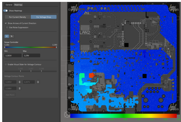
Hình 4.71: Biểu đồ phân bố điện áp trên nguồn +3V3.
