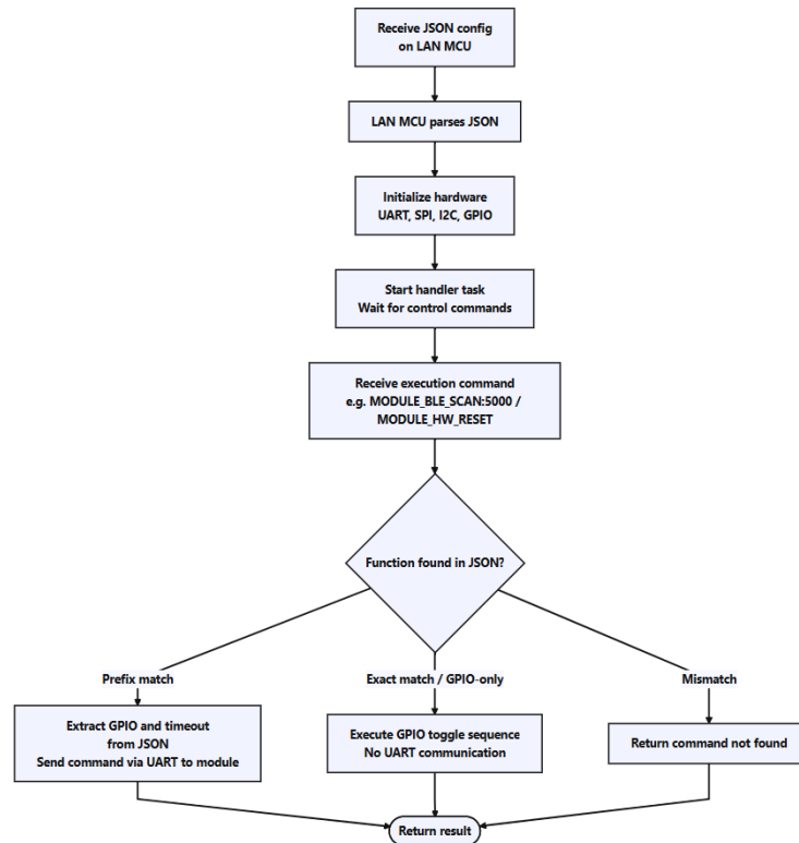
Hình 4.54: Luồng hoạt động của Module Base Setting
