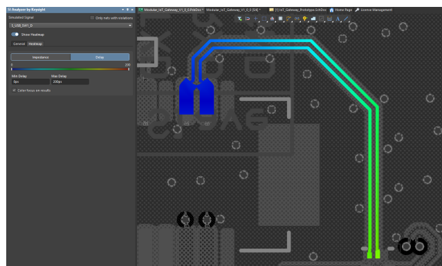
Hình 4.60: Biểu đồ phân bố độ trễ lan truyền (Propagation Delay) đường vi sai.
