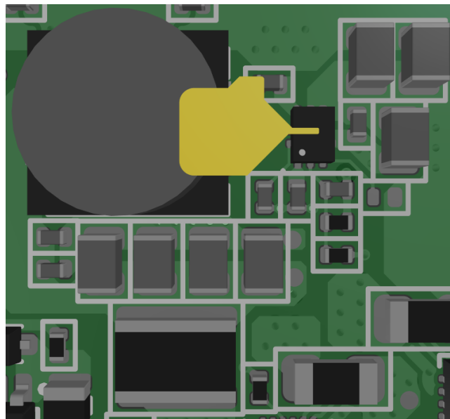
Hình 4.44: Điểm chuyển mạch trong nguồn xung +3V3.
