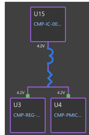
Hình 4.63: Cây phân phối nguồn +4V2_VSYS.
