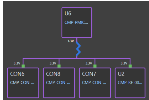
Hình 4.72: Cây phân phối nguồn +3V3_CTRL.
