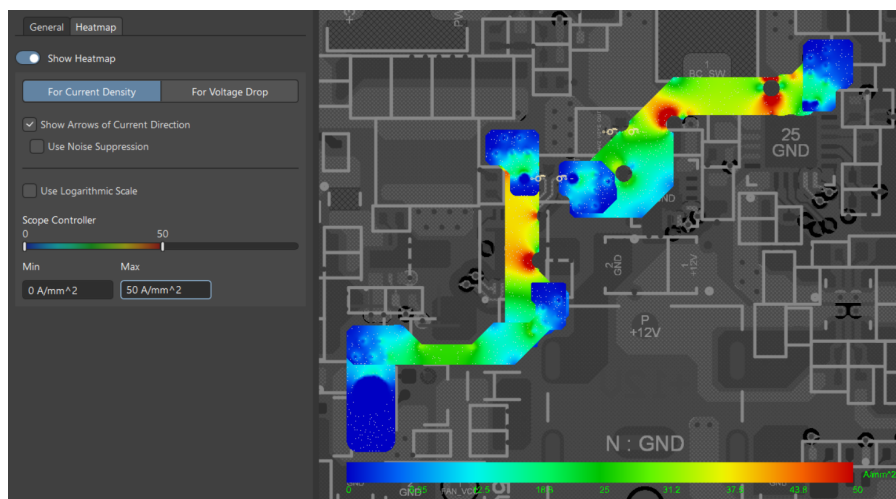
Hình 4.76: Biểu đồ phân bố mật độ dòng điện của nguồn +3V7_VBAT.
