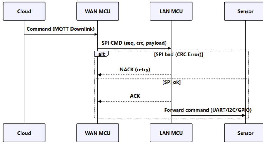
Hình 4.4: Sequence diagram: luồng xử lý dữ liệu end-to-end downlink
