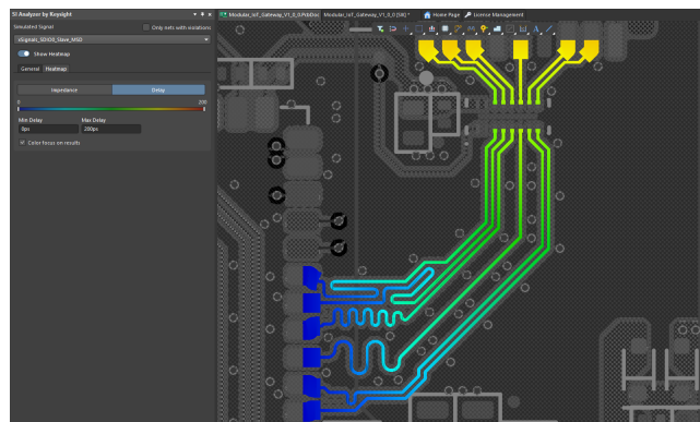
Hình 4.57: Biểu đồ phân bố độ trễ lan truyền (Propagation Delay) đường tín hiệu đơn cực.
