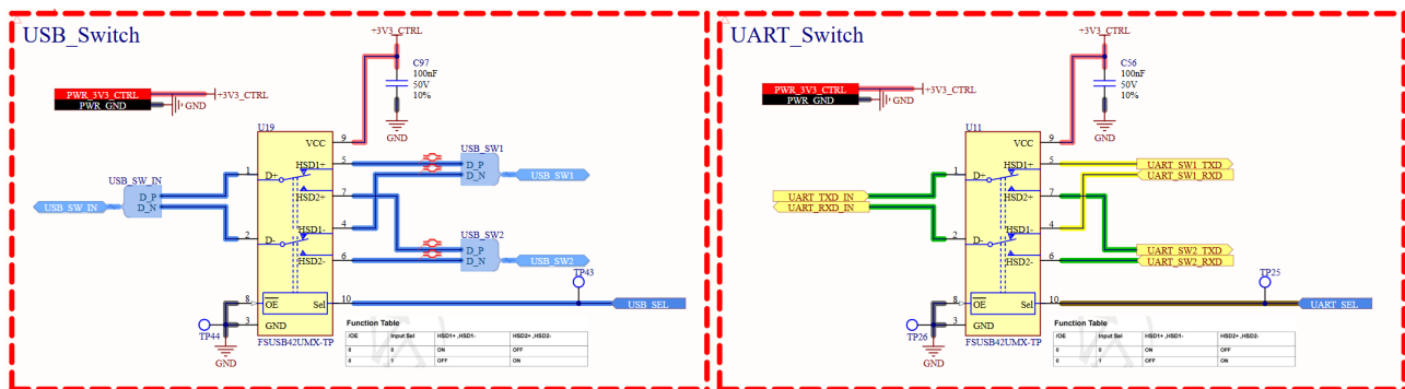
Hình 4.25: Sơ đồ nguyên lý mạch USB/UART Switch
