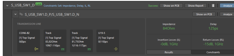
Hình 4.61: Bảng tổng hợp thông số mô phỏng đường vi sai.
