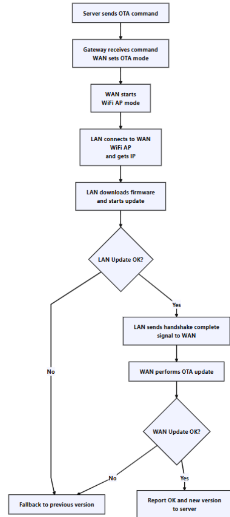
Hình 4.53: Lưu đồ giải thuật FOTA cho Dual-MCU Gateway
