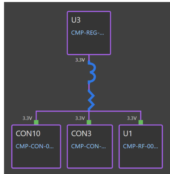
Hình 4.69: Cây phân phối nguồn +3V3.
