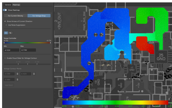
Hình 4.65: Biểu đồ phân bố điện áp trên nguồn +4V2_VSYS.
