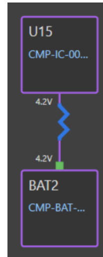
Hình 4.75: Cây phân phối nguồn +3V7_VBAT.
