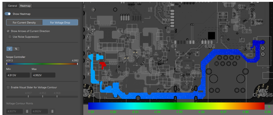
Hình 4.68: Biểu đồ phân bố điện áp trên nguồn +5V0_CTRL.
