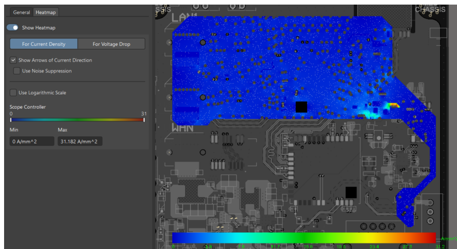
Hình 4.73: Biểu đồ phân bố mật độ dòng điện của nguồn +3V3_CTRL.
