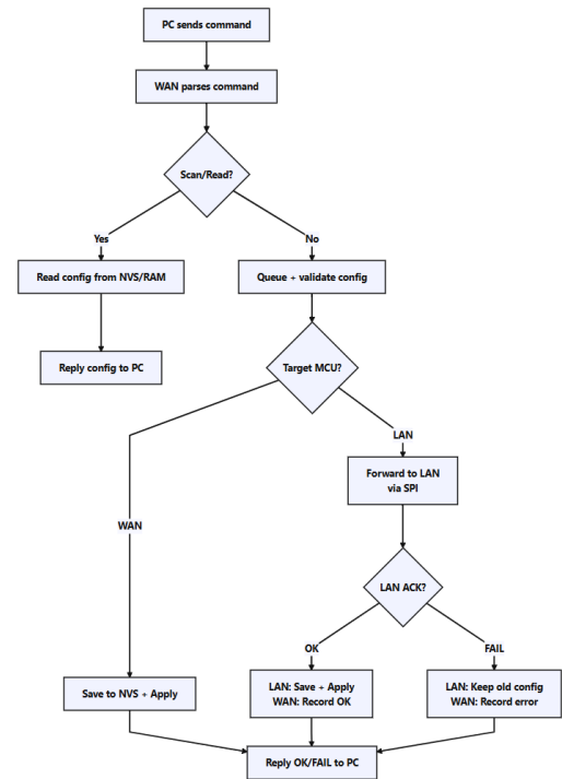
Hình 4.51: Lưu đồ giải thuật Data Communication Handler – giao tiếp cấu hình qua USB/UART
