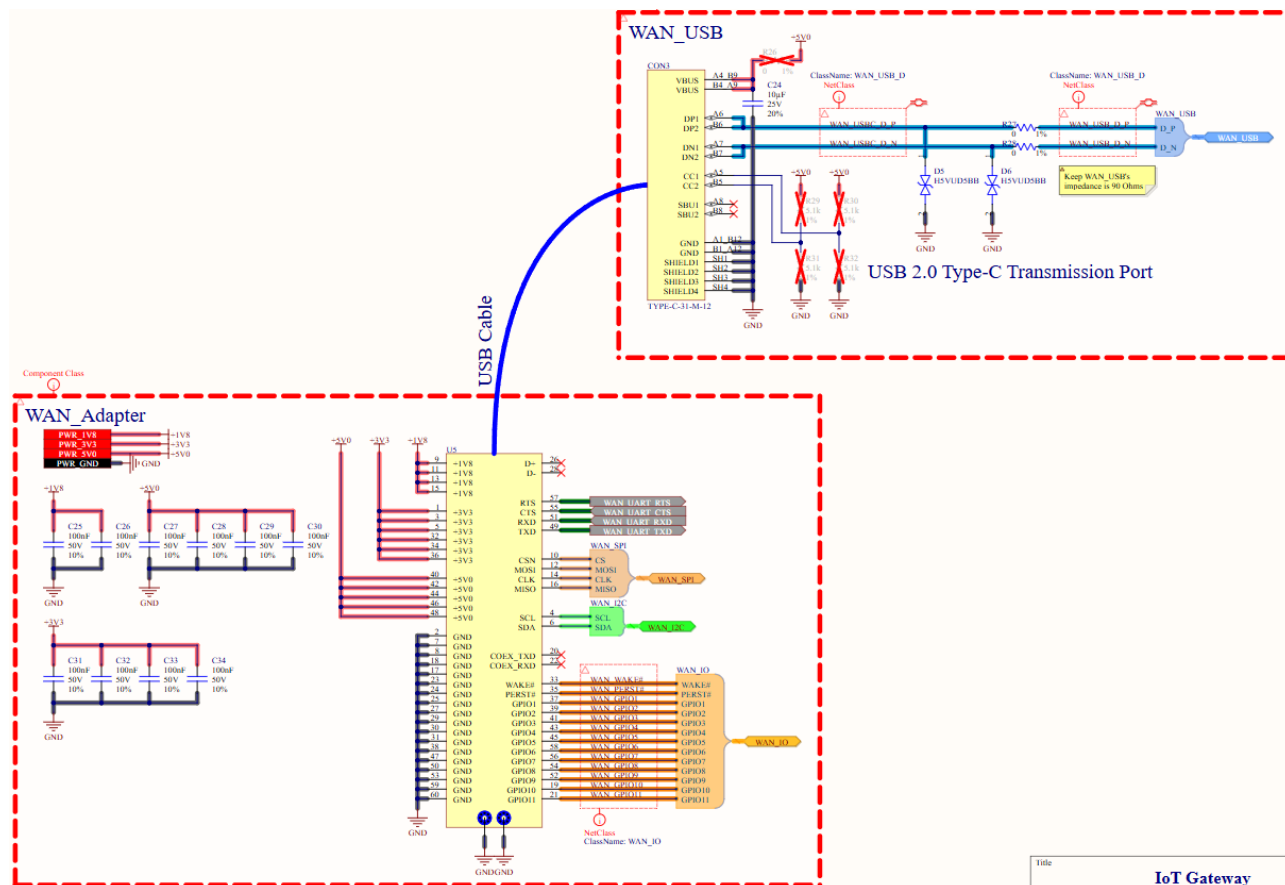
Hình 4.17: Sơ đồ nguyên lý mạch WAN
