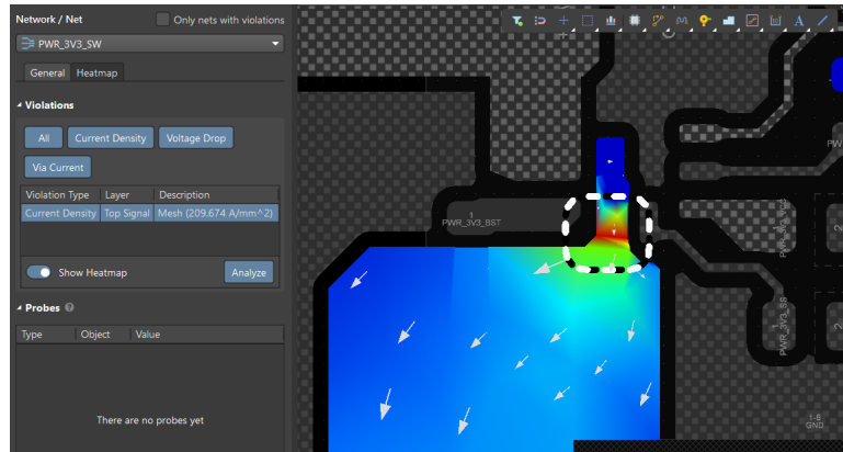
Hình 4.68: Mật độ dòng điện cao đột biến tại pinout nguồn xung +3V3.
