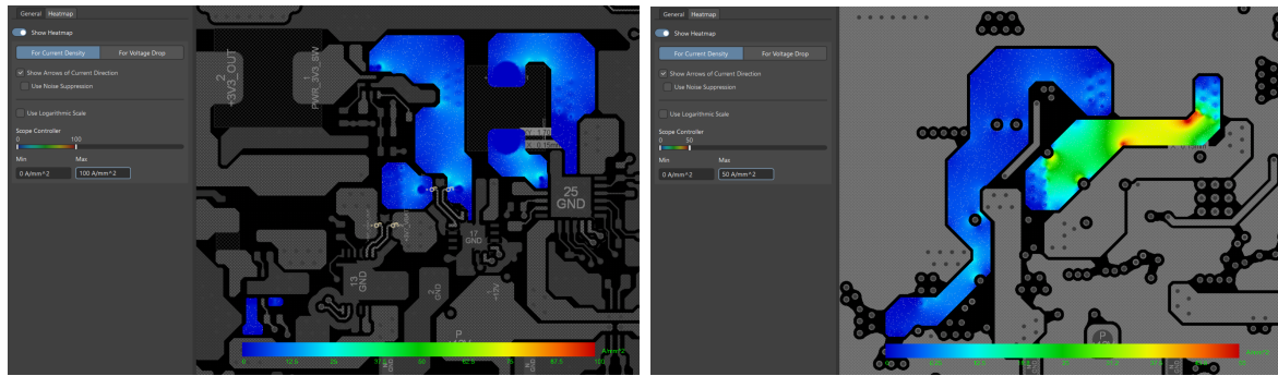
Hình 4.60: Biểu đồ phân bố mật độ dòng điện của nguồn +4V2_VSYS.
