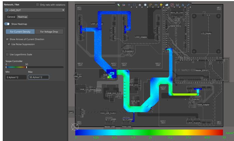
Hình 4.66: Biểu đồ phân bố mật độ dòng điện (Current Density Heatmap) trên nguồn +5V0.
