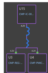
Hình 4.59: Cây phân phối nguồn +4V2_VSYS.
