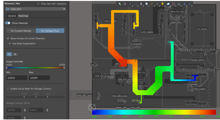
Hình 4.62: Biểu đồ phân bố điện áp (Voltage Drop Heatmap) trên nguồn +5V0.
