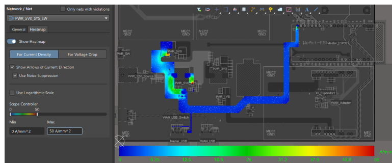
Hình 4.64: Biểu đồ phân bố mật độ dòng điện (Current Density Heatmap) trên nguồn +5V0_SYS.
