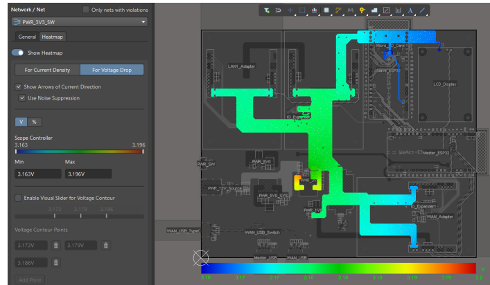
Hình 4.63: Biểu đồ phân bố điện áp (Voltage Drop Heatmap) trên nguồn +3V3.
