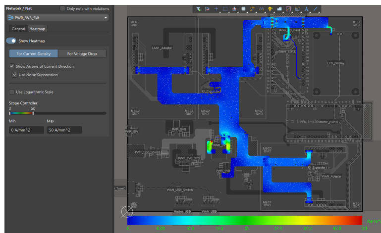
Hình 4.67: Biểu đồ phân bố mật độ dòng điện (Current Density Heatmap) trên nguồn +3V3.
