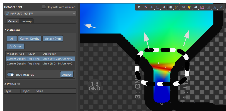
Hình 4.65: Mật độ dòng điện cao đột biến tại pinout nguồn xung +5V0_SYS.
