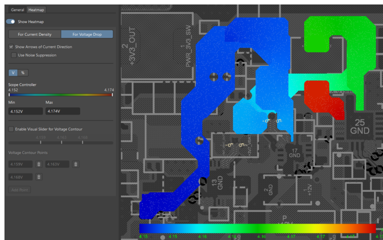
Hình 4.61: Biểu đồ phân bố điện áp (Voltage Drop Heatmap) trên nguồn +4V2_VSYS.
