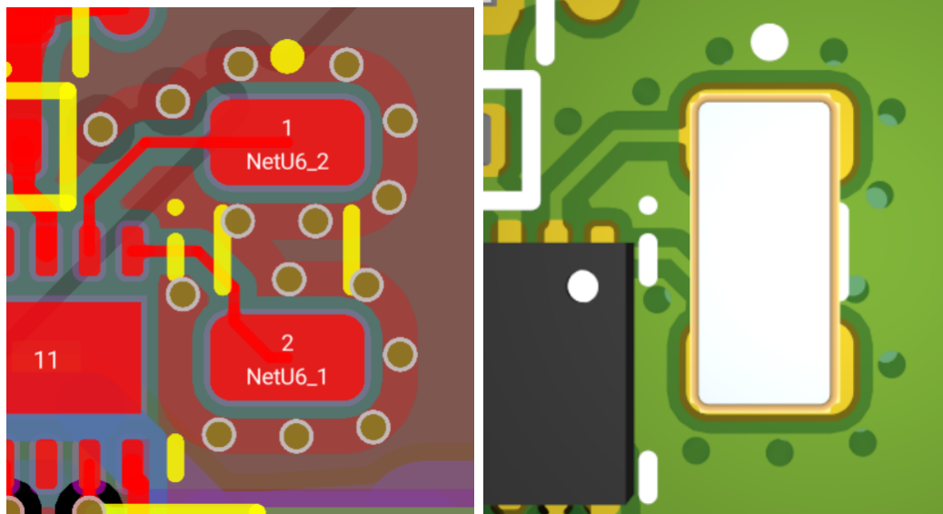
Hình 4.38: Kỹ thuật tạo vòng bảo vệ (Guard Ring) và via stitching xung quanh khối thạch anh để cô lập nhiễu.
