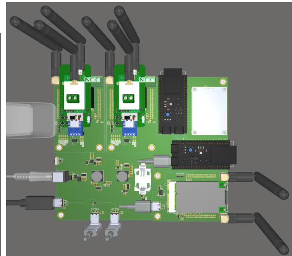
Hình 4.37: Sơ đồ quy hoạch phân vùng chức năng trên PCB (Floor-planning)
