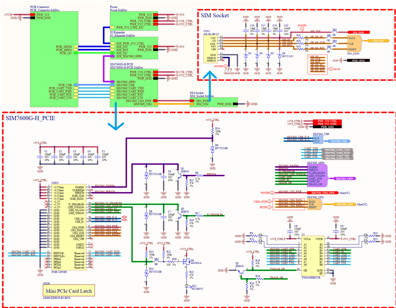
Hình 4.31: Sơ đồ nguyên lý mạch WAN Adapter
