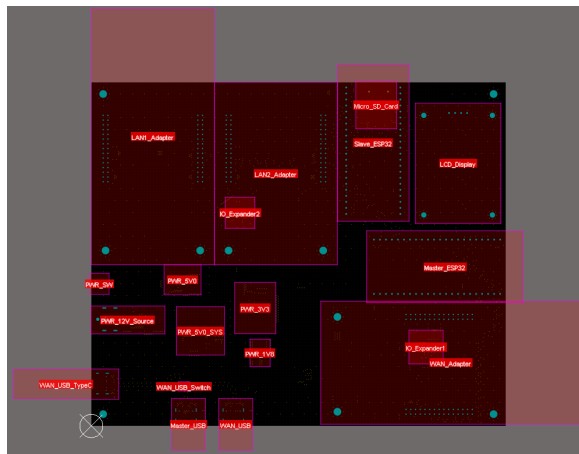
Hình 4.37: Sơ đồ quy hoạch phân vùng chức năng trên PCB (Floor-planning)
