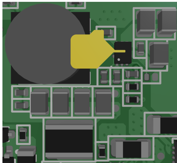
Hình 4.44: Điểm chuyển mạch trong nguồn xung +3V3.
