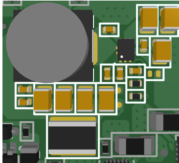
Hình 4.43: Vị trí các tụ điện trong nguồn xung +3V3.
