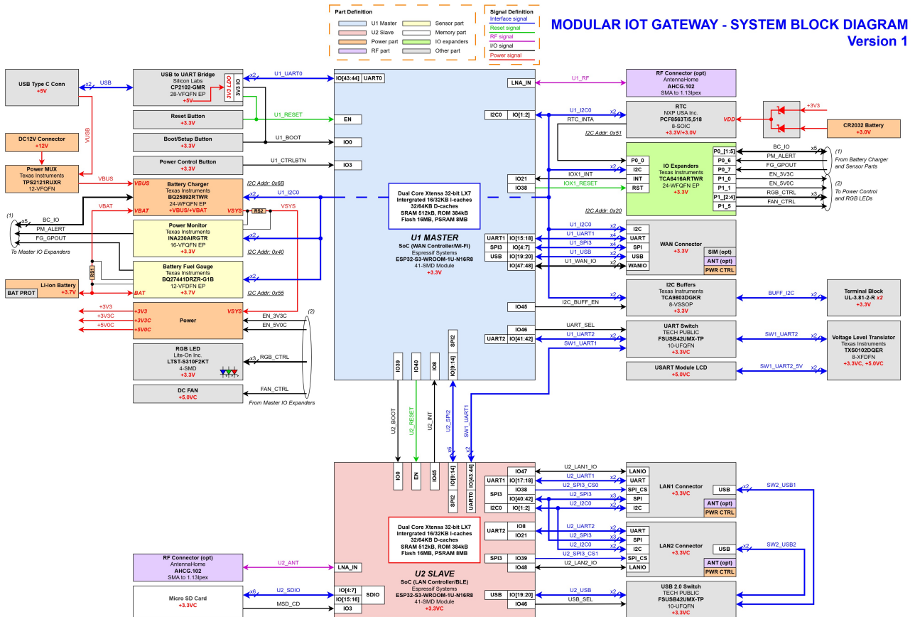
Hình 4.8: Sơ đồ khối hệ thống
