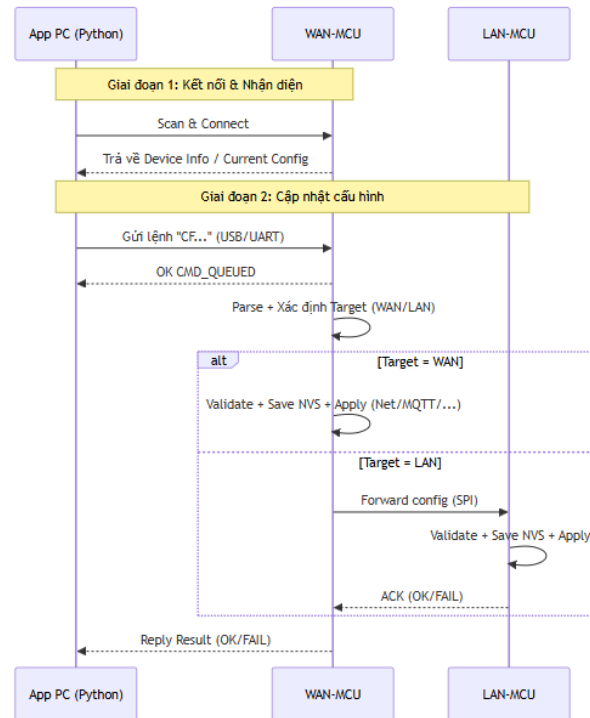
Hình 4.6: Sequence diagram: cập nhật cấu hình từ App PC
