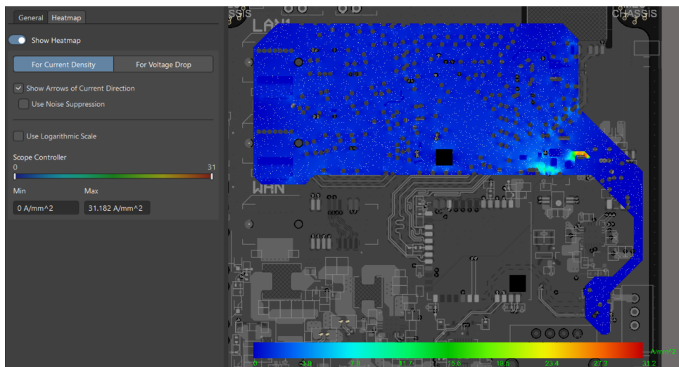
Hình 4.71: Biểu đồ phân bố mật độ dòng điện của nguồn +3V3_CTRL.
