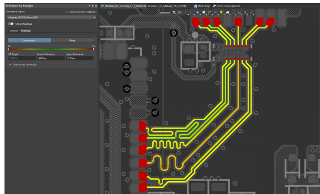
Hình 4.54: Biểu đồ phân bố trở kháng (Impedance Heatmap) đường tín hiệu đơn cực.
