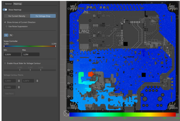
Hình 4.69: Biểu đồ phân bố điện áp trên nguồn +3V3.
