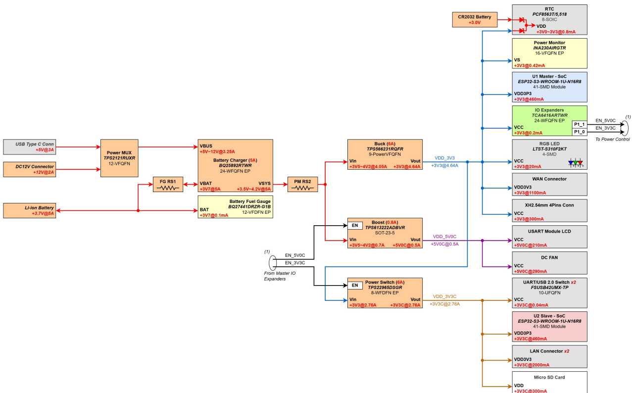
Hình 4.9: Sơ đồ hệ thống nguồn
