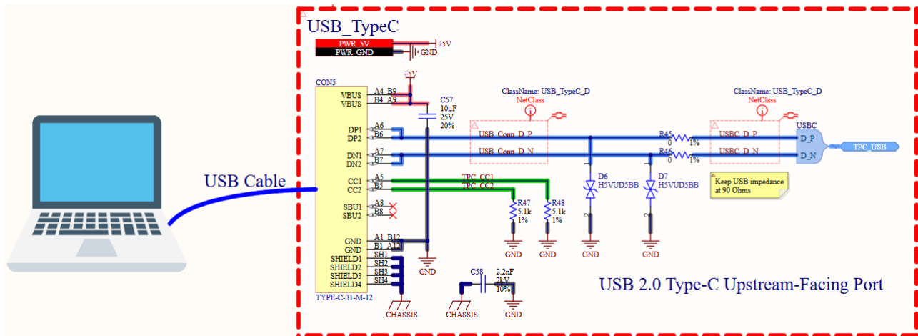
Hình 4.18: Sơ đồ nguyên lý mạch USB
