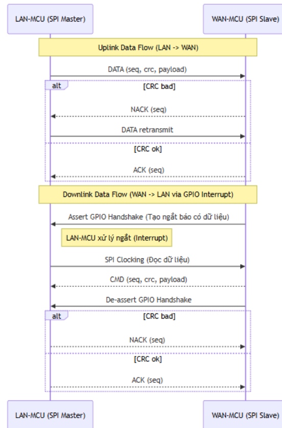
Hình 4.5: Sequence diagram: giao tiếp LAN-MCU ↔ WAN-MCU qua SPI
