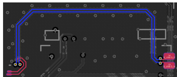
Hình 4.47: Định tuyến USB.
