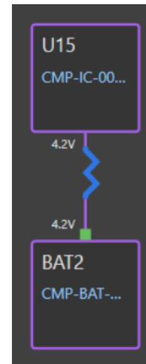
Hình 4.73: Cây phân phối nguồn +3V7_VBAT.
