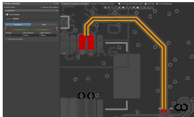
Hình 4.57: Biểu đồ phân bố trở kháng (Impedance Heatmap) đường vi sai.
