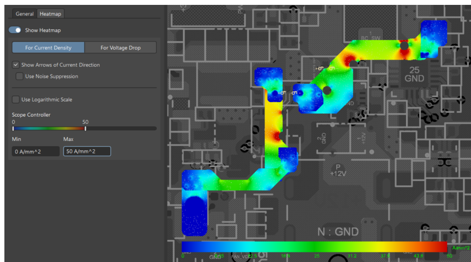
Hình 4.74: Biểu đồ phân bố mật độ dòng điện của nguồn +3V7_VBAT.
