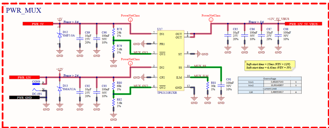
Hình 4.15: Sơ đồ nguyên lý mạch Power MUX
