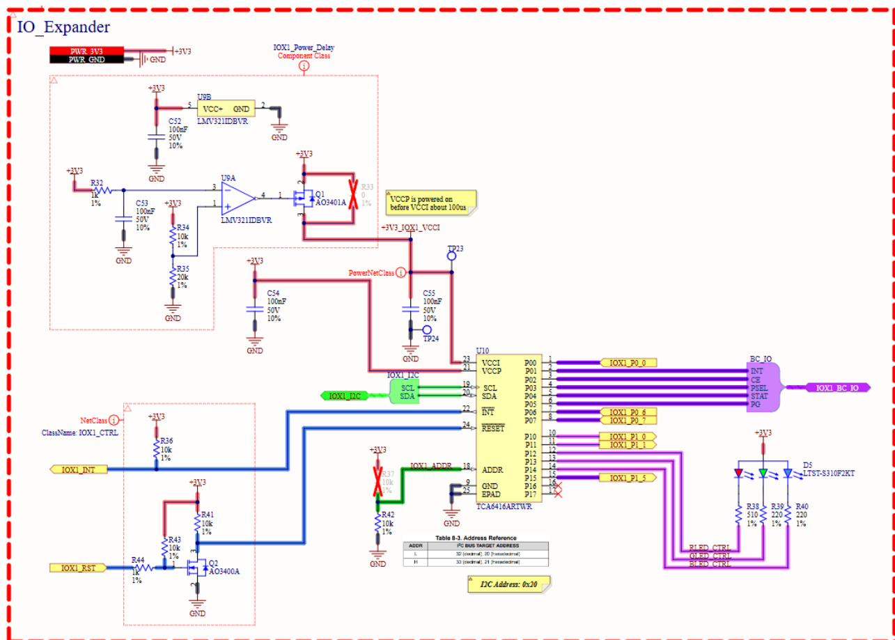
Hình 4.20: Sơ đồ nguyên lý mạch IO Expanders
