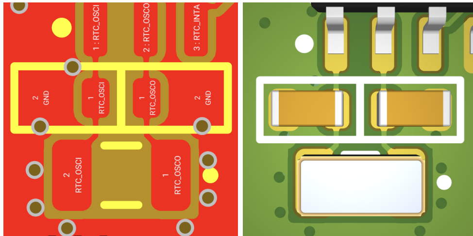
Hình 4.40: Kỹ thuật tạo Guard Ring và via stitching xung quanh khối thạch anh để cô lập nhiễu.
