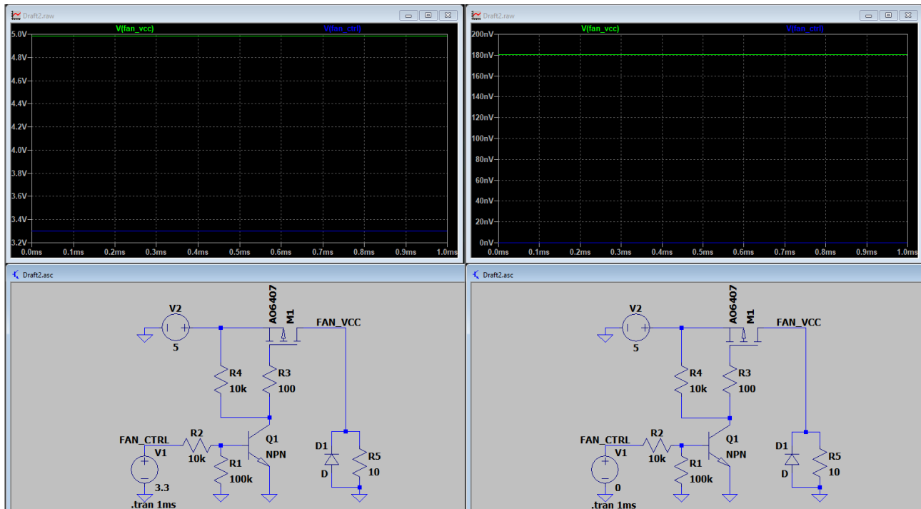
Hình 4.30: Thực hiện mô phỏng mạch điều khiển quạt DC trên LTspice
