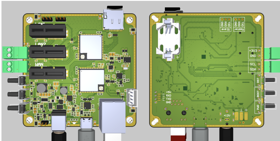
Hình 4.39: Sơ đồ quy hoạch phân vùng chức năng trên PCB (Floor-planning).
