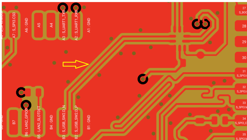
Hình 4.41: Kỹ thuật bọc mass và stitching via dọc theo đường tín hiệu USB tốc độ cao.
