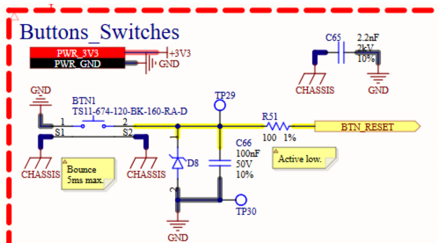
Hình 4.28: Sơ đồ nguyên lý mạch nút nhấn
