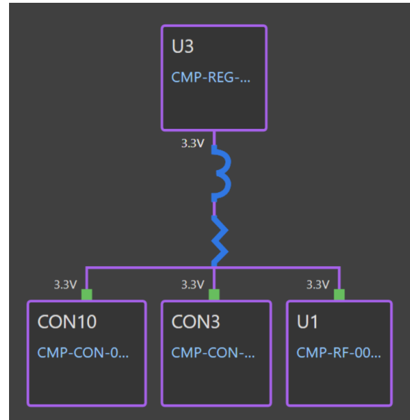
Hình 4.67: Cây phân phối nguồn +3V3.
