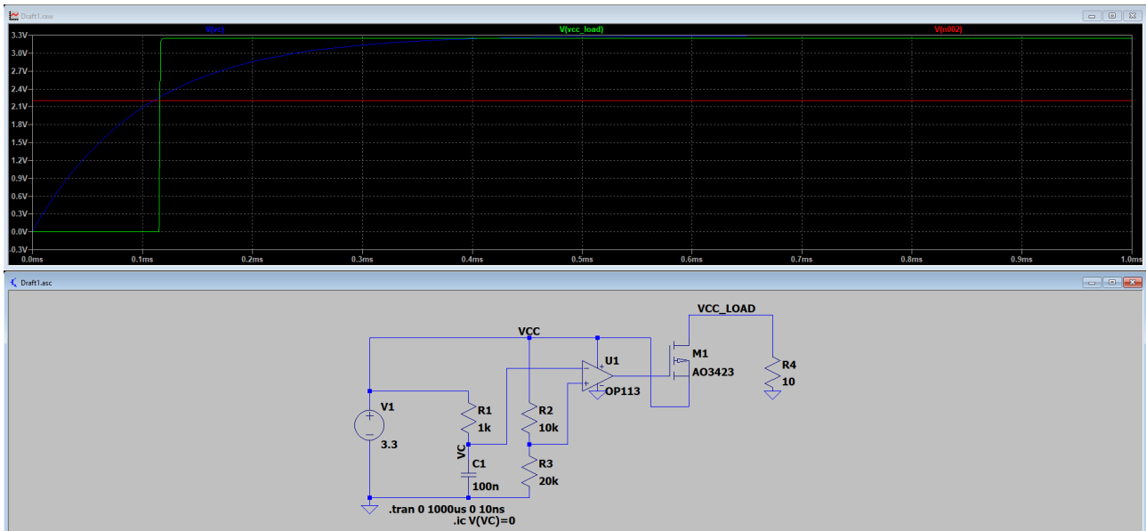
Hình 4.22: Kết quả mô phỏng mạch delay khởi động nguồn VCCI cho IO Expander
