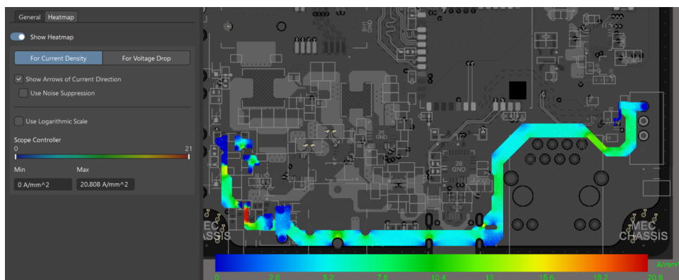
Hình 4.65: Biểu đồ phân bố mật độ dòng điện của nguồn +5V0_CTRL.
