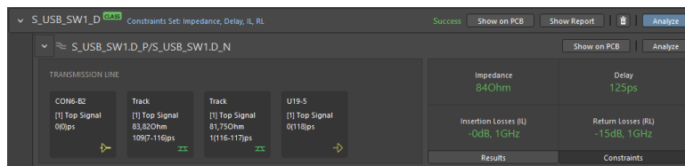
Hình 4.59: Bảng tổng hợp thông số mô phỏng đường vi sai.
