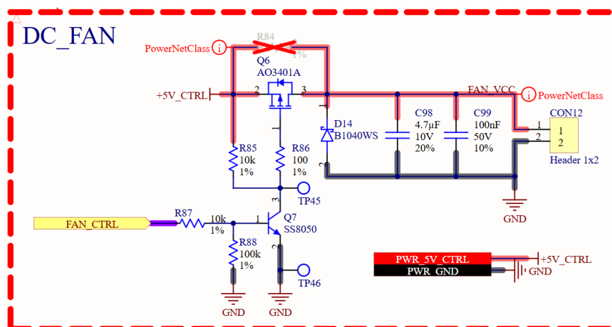
Hình 4.29: Sơ đồ nguyên lý mạch điều khiển quạt DC
