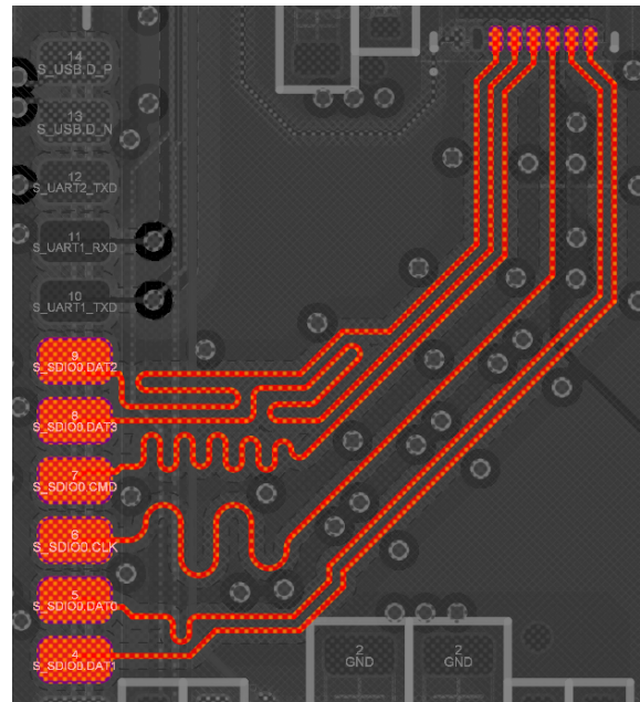
Hình 4.48: Định tuyến SDIO giữa ESP32-S3 Slave với Micro SD Card.
