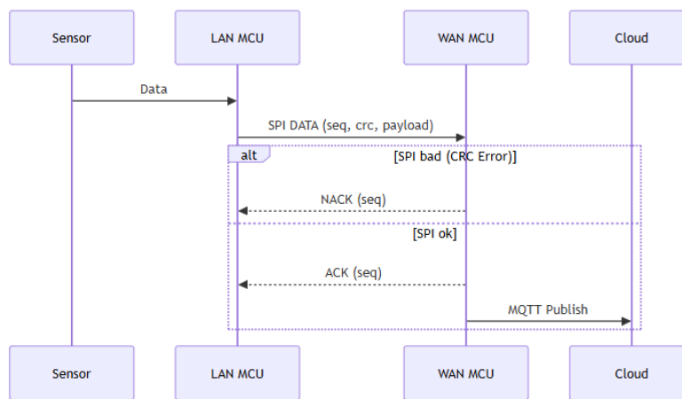
Hình 4.3: Sequence diagram: luồng xử lý dữ liệu end-to-end uplink
