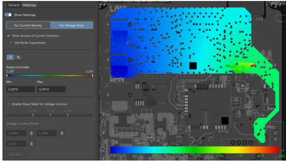
Hình 4.72: Biểu đồ phân bố điện áp trên nguồn +3V3_CTRL.
