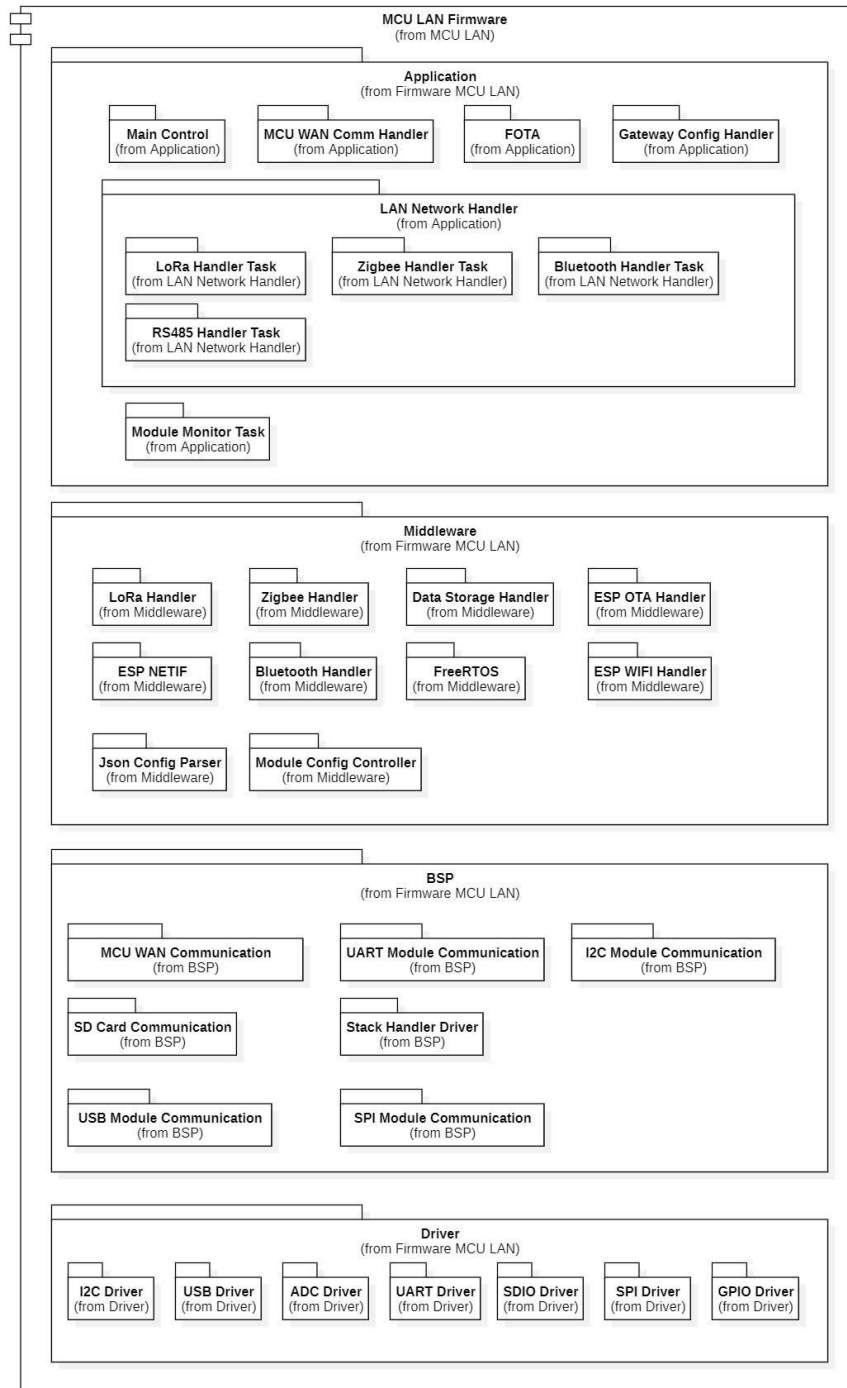
Hình 4.49: MCU LAN Firmware
