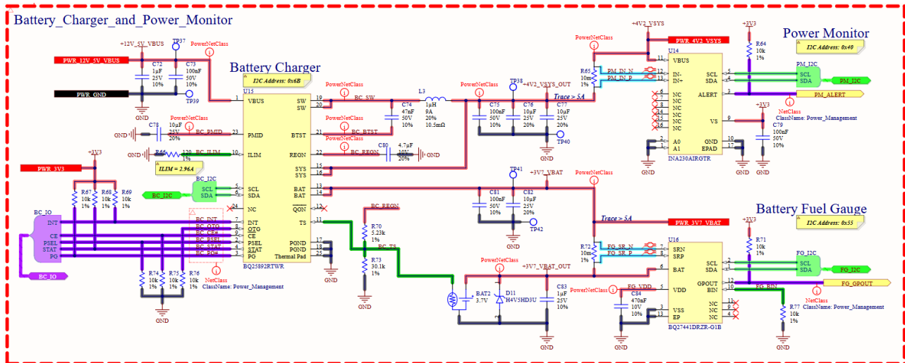
Hình 4.16: Sơ đồ nguyên lý mạch sạc, quản lý pin LiPo và giám sát công suất
