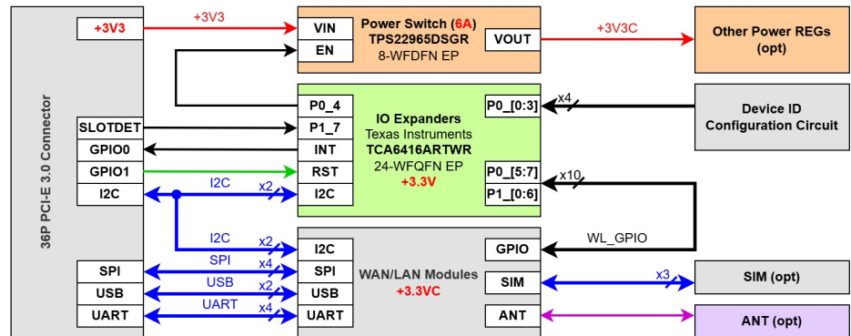
Hình 4.10: Sơ đồ khối mạch adapter
