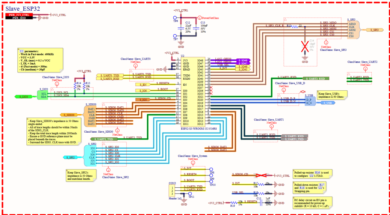
Hình 4.13: Sơ đồ nguyên lý ESP32 Slave
