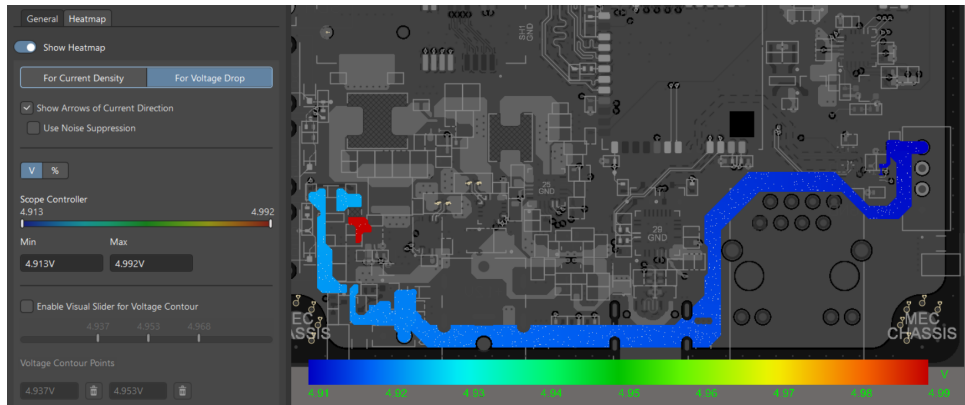
Hình 4.66: Biểu đồ phân bố điện áp trên nguồn +5V0_CTRL.
