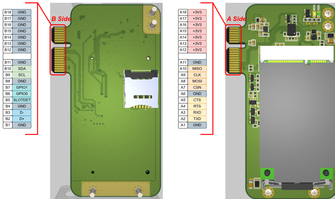
Hình 4.2: Sơ đồ chân Module Adapter
