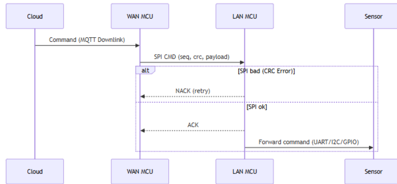
Hình 4.4: Sequence diagram: luồng xử lý dữ liệu end-to-end downlink
