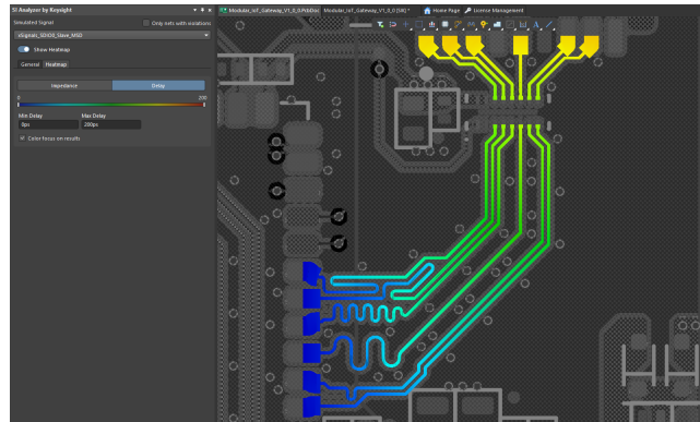
Hình 4.55: Biểu đồ phân bố độ trễ lan truyền (Propagation Delay) đường tín hiệu đơn cực.
