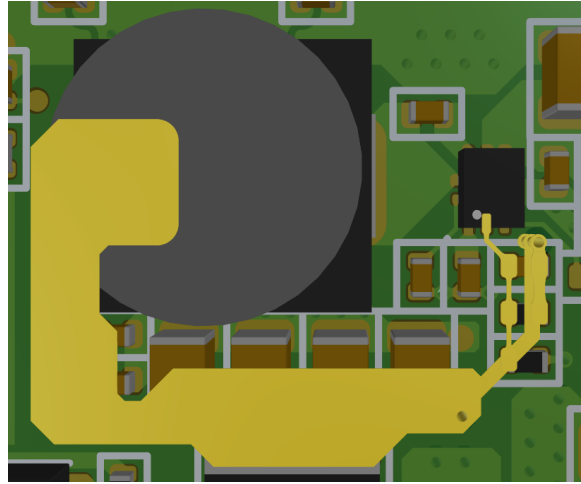
Hình 4.45: Định tuyến hồi tiếp trong nguồn xung +3V3.
