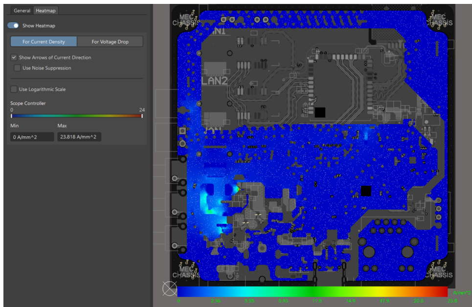
Hình 4.68: Biểu đồ phân bố mật độ dòng điện của nguồn +3V3.
