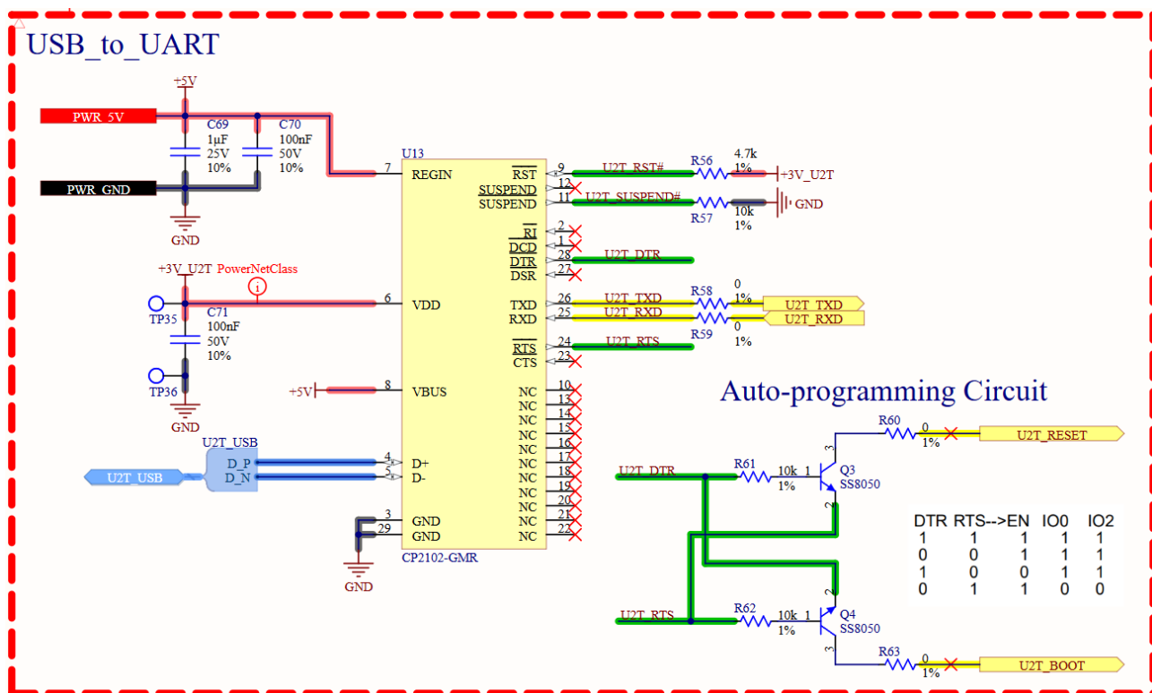
Hình 4.19: Sơ đồ nguyên lý mạch USB to UART Bridge
