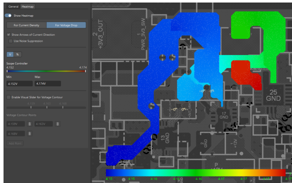
Hình 4.63: Biểu đồ phân bố điện áp trên nguồn +4V2_VSYS.
