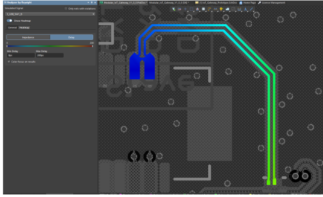
Hình 4.58: Biểu đồ phân bố độ trễ lan truyền (Propagation Delay) đường vi sai.
