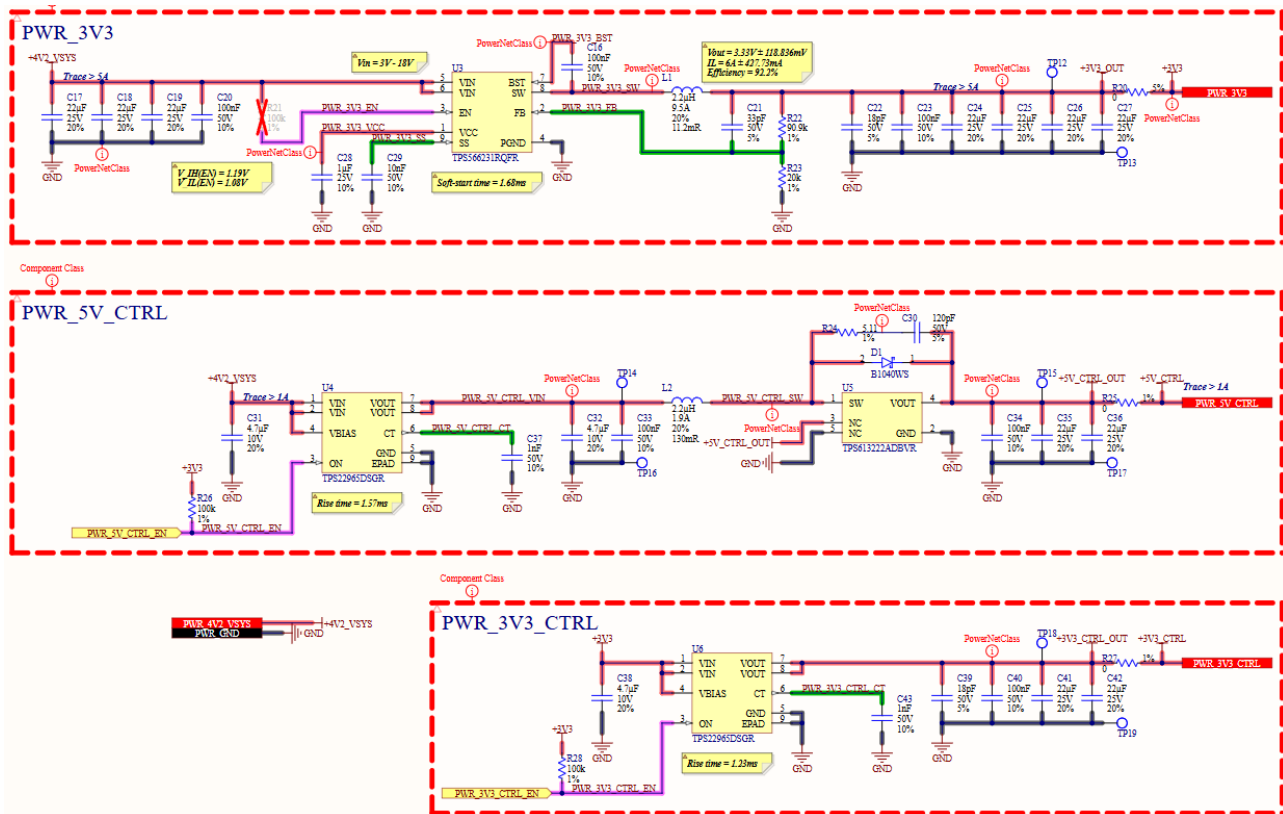
Hình 4.17: Sơ đồ nguyên lý mạch nguồn DC-DC
