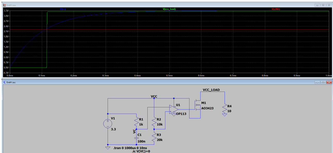
Hình 4.14: Kết quả mô phỏng mạch delay khởi động nguồn VCCI cho IO Expander
