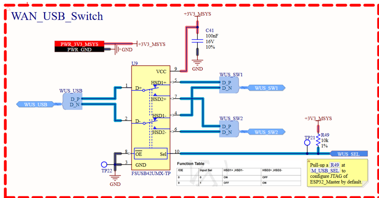
Hình 4.11: Sơ đồ nguyên lý mạch USB Switch
