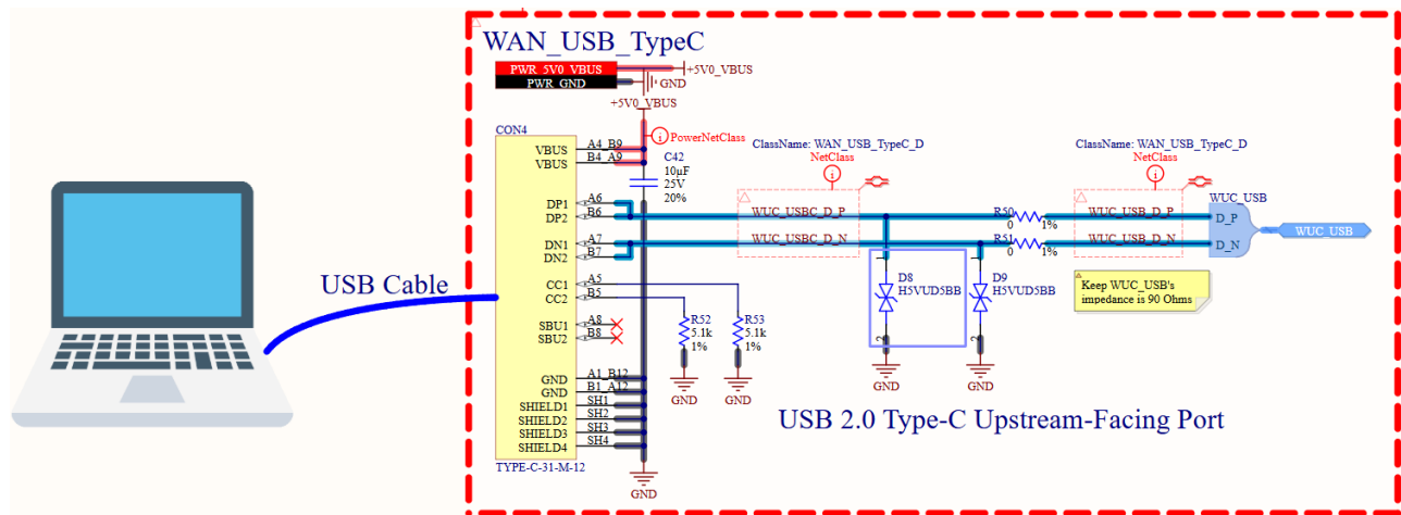
Hình 4.10: Sơ đồ nguyên lý mạch USB
