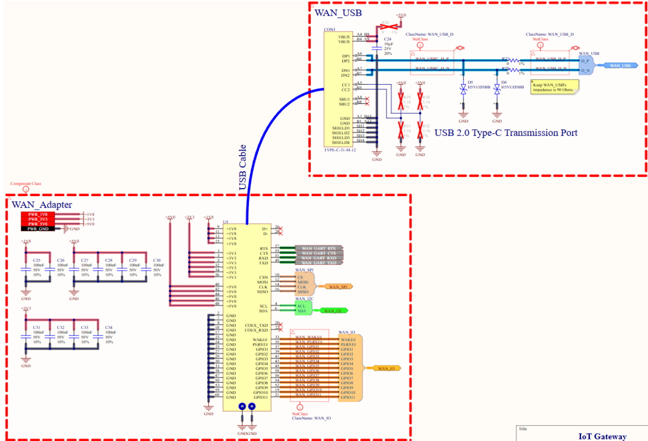
Hình 4.17: Sơ đồ nguyên lý mạch WAN
