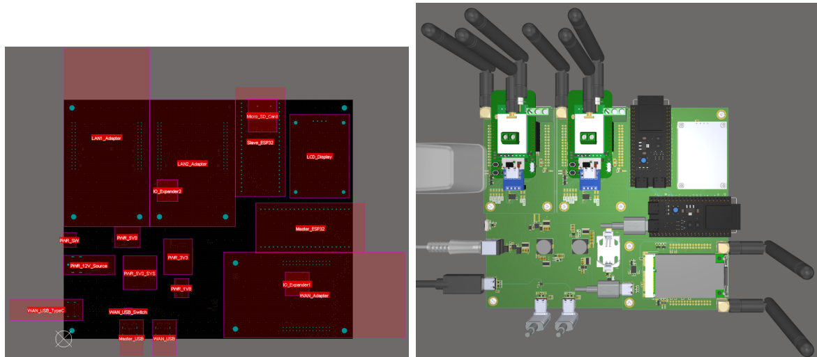
Hình 4.24: Sơ đồ quy hoạch phân vùng chức năng trên PCB (Floor-planning)
