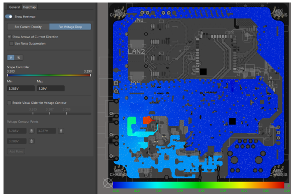
Hình 4.68: Biểu đồ phân bố điện áp trên nguồn +3V3.
