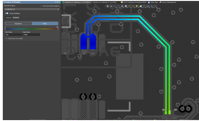
Hình 4.57: Biểu đồ phân bố độ trễ lan truyền (Propagation Delay) đường vi sai.
