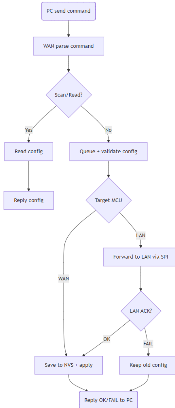
Hình 4.51: Lưu đồ giải thuật Data Communication Handler – giao tiếp cấu hình qua USB/UART
