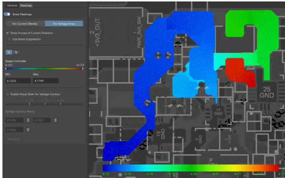
Hình 4.62: Biểu đồ phân bố điện áp trên nguồn +4V2_VSYS.
