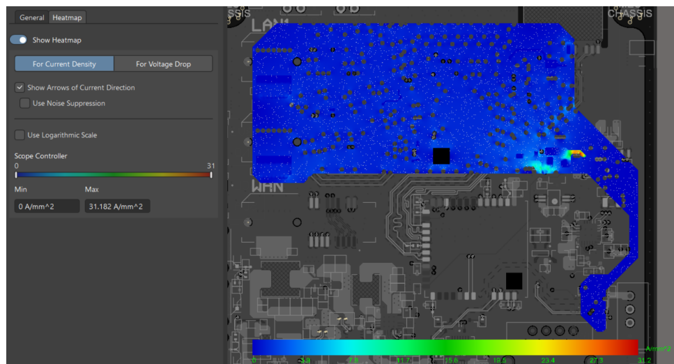
Hình 4.70: Biểu đồ phân bố mật độ dòng điện của nguồn +3V3_CTRL.
