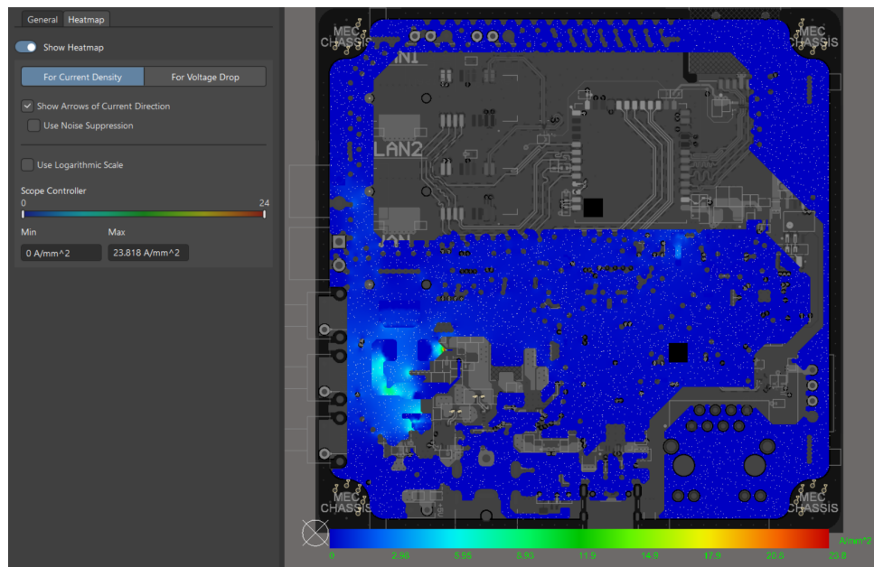
Hình 4.67: Biểu đồ phân bố mật độ dòng điện của nguồn +3V3.
