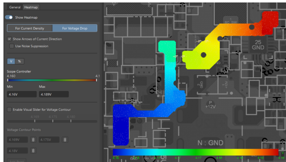
Hình 4.74: Biểu đồ phân bố điện áp trên nguồn +3V7_VBAT.
