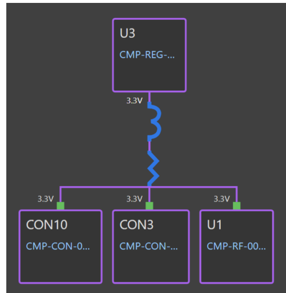
Hình 4.66: Cây phân phối nguồn +3V3.
