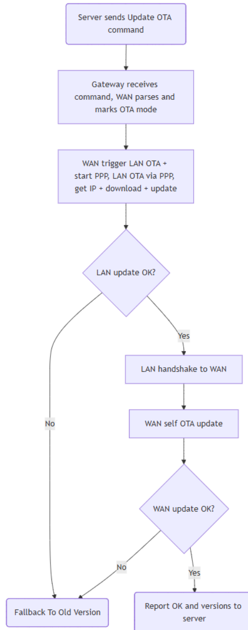
Hình 4.52: Lưu đồ giải thuật FOTA cho Dual-MCU Gateway
