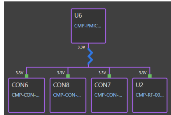
Hình 4.69: Cây phân phối nguồn +3V3_CTRL.
