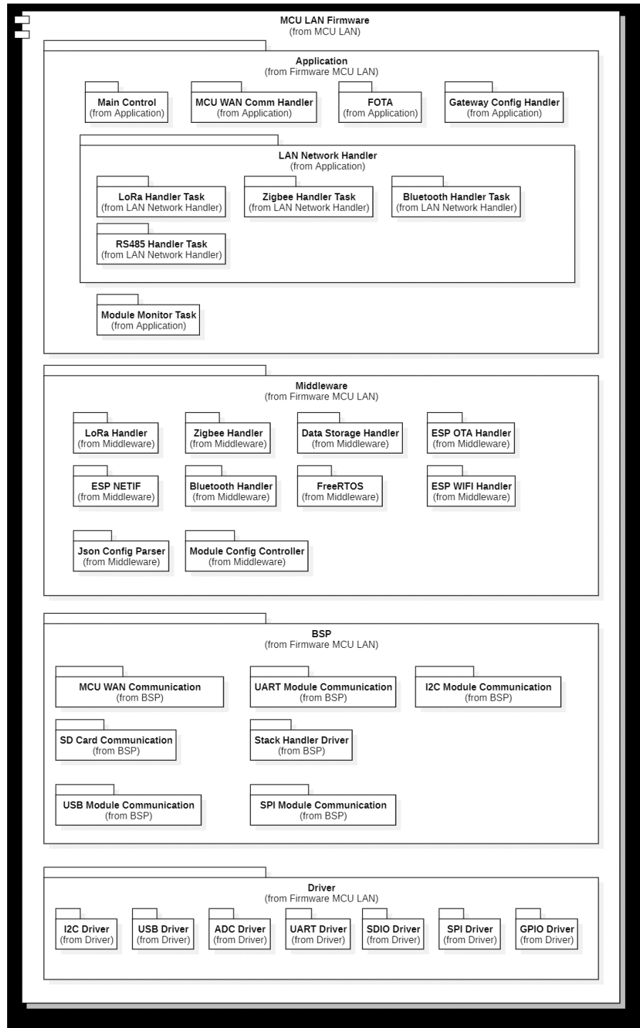
Hình 4.49: MCU LAN Firmware
