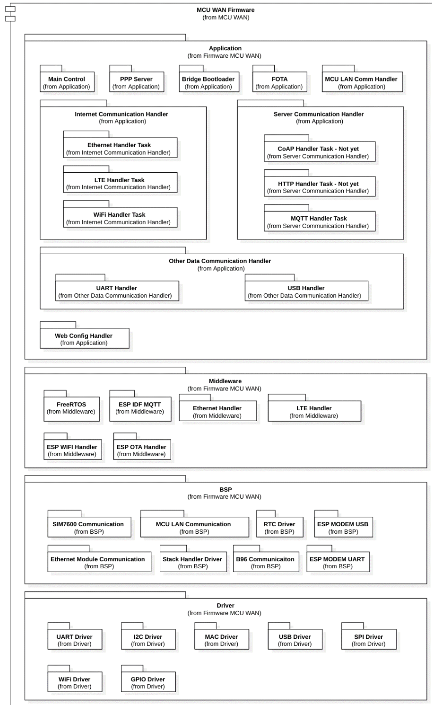
Hình 4.50: MCU WAN Firmware
