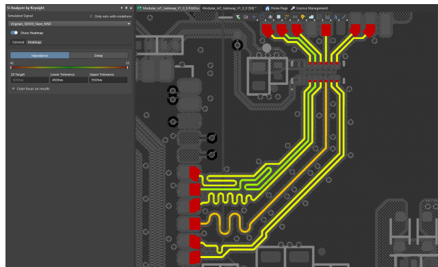
Hình 4.53: Biểu đồ phân bố trở kháng (Impedance Heatmap) đường tín hiệu đơn cực.
