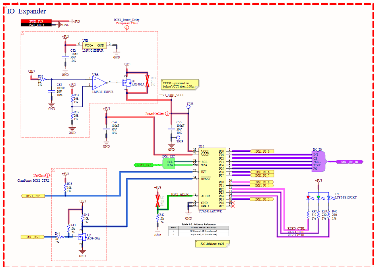
Hình 4.20: Sơ đồ nguyên lý mạch IO Expanders
