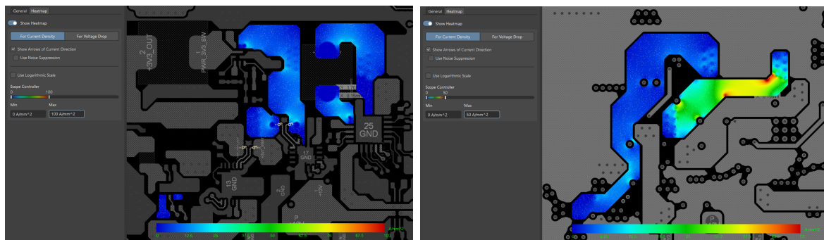
Hình 4.61: Biểu đồ phân bố mật độ dòng điện của nguồn +4V2_VSYS.
