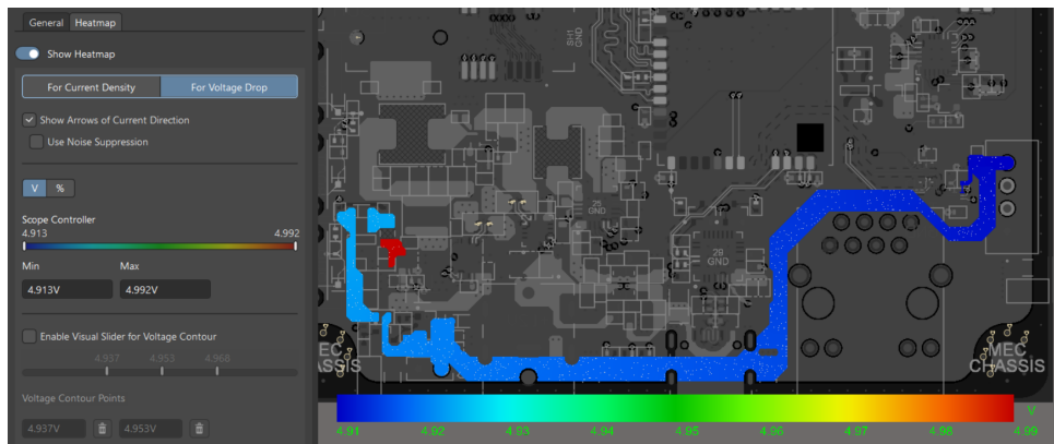
Hình 4.65: Biểu đồ phân bố điện áp trên nguồn +5V0_CTRL.
