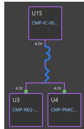
Hình 4.60: Cây phân phối nguồn +4V2_VSYS.
