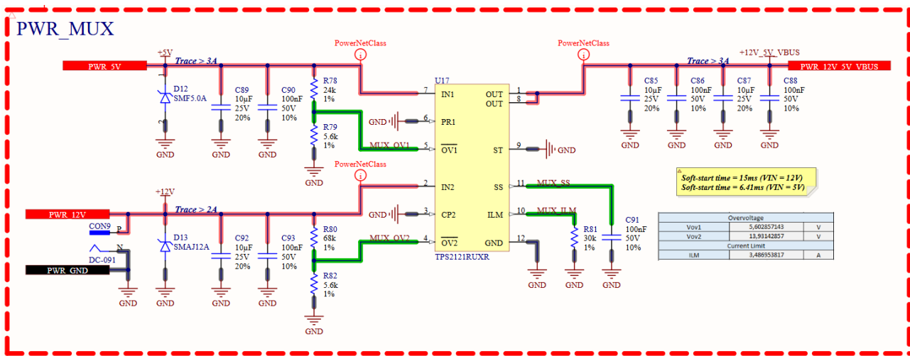
Hình 4.15: Sơ đồ nguyên lý mạch Power MUX
