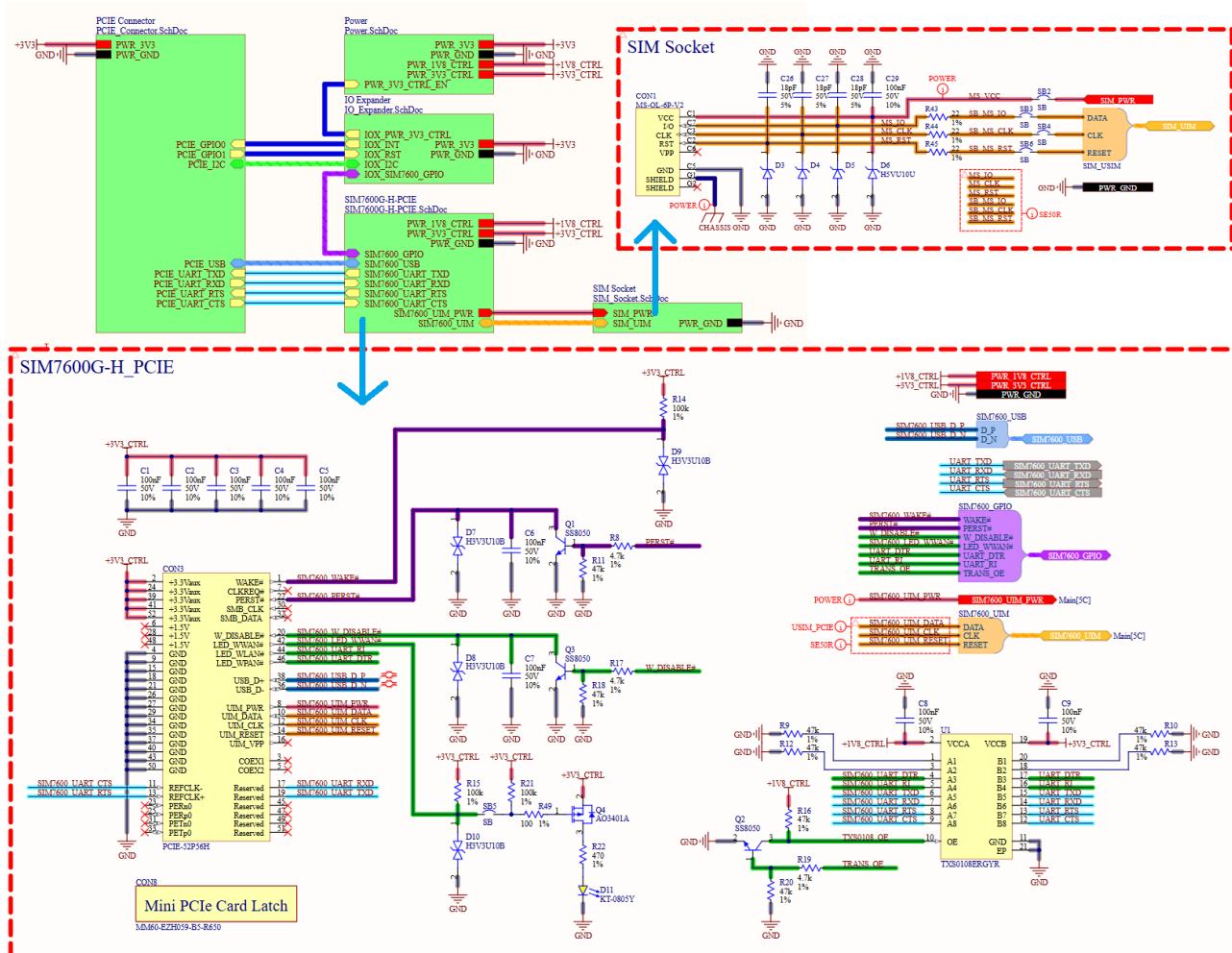
Hình 4.32: Sơ đồ nguyên lý mạch WAN Adapter LTE
