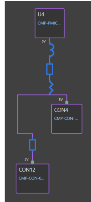
Hình 4.63: Cây phân phối nguồn +5V0_CTRL.
