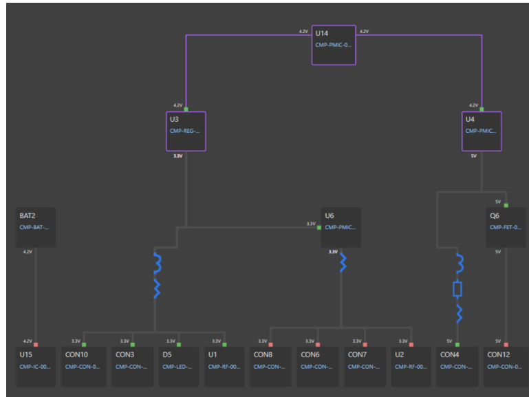
Hình 4.59: Cấu trúc mạng phân phối nguồn.
