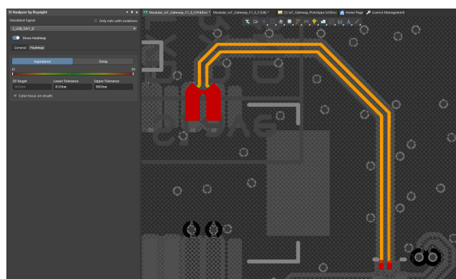
Hình 4.56: Biểu đồ phân bố trở kháng (Impedance Heatmap) đường vi sai.
