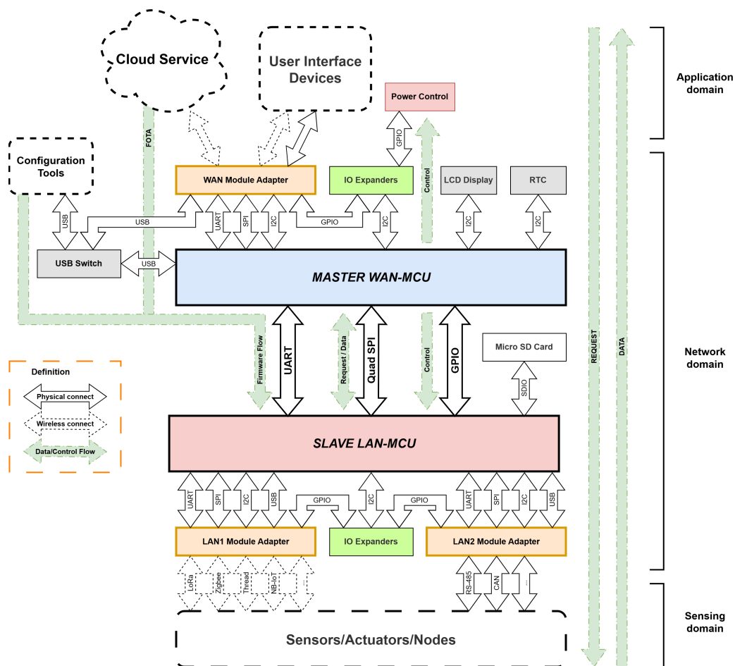
Hình 4.1: Sơ đồ khối Hệ thống
