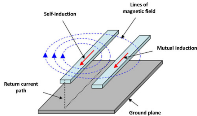
Hình 3.6: Minh họa hiện tượng nhiễu xuyên kênh giữa các đường truyền đặt gần nhau
