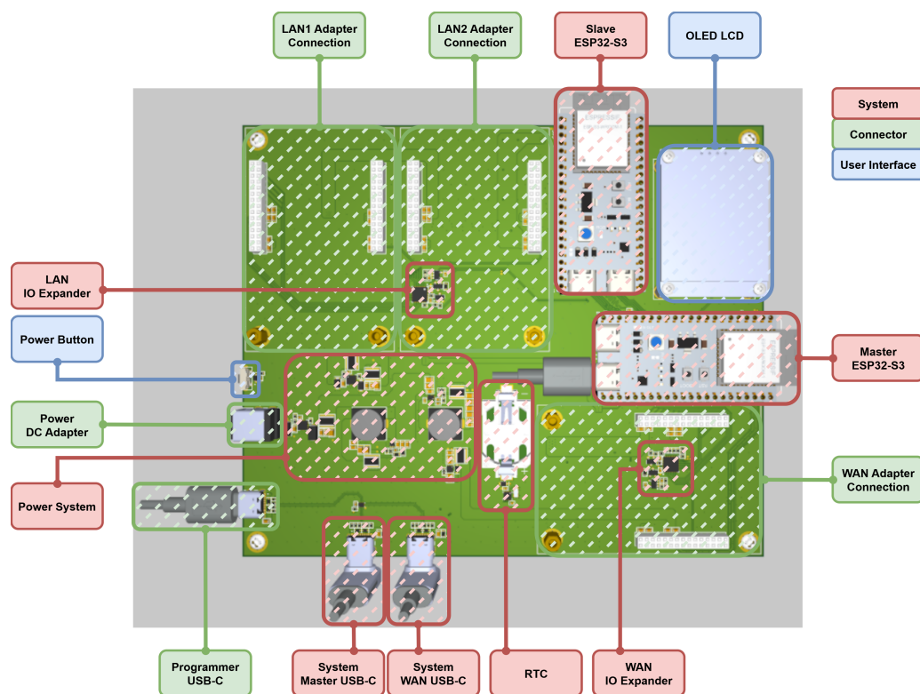
Hình 6.1: Assembly Diagram.
