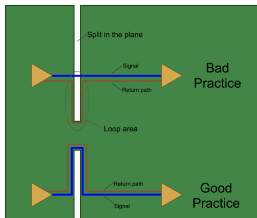
Hình 3.4: Minh hoạ return path liên tục dưới trace trên mặt phẳng tham chiếu
