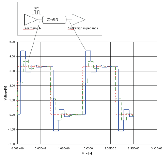
Hình 3.3: Minh hoạ hiện tượng ringing do không khớp trở kháng
