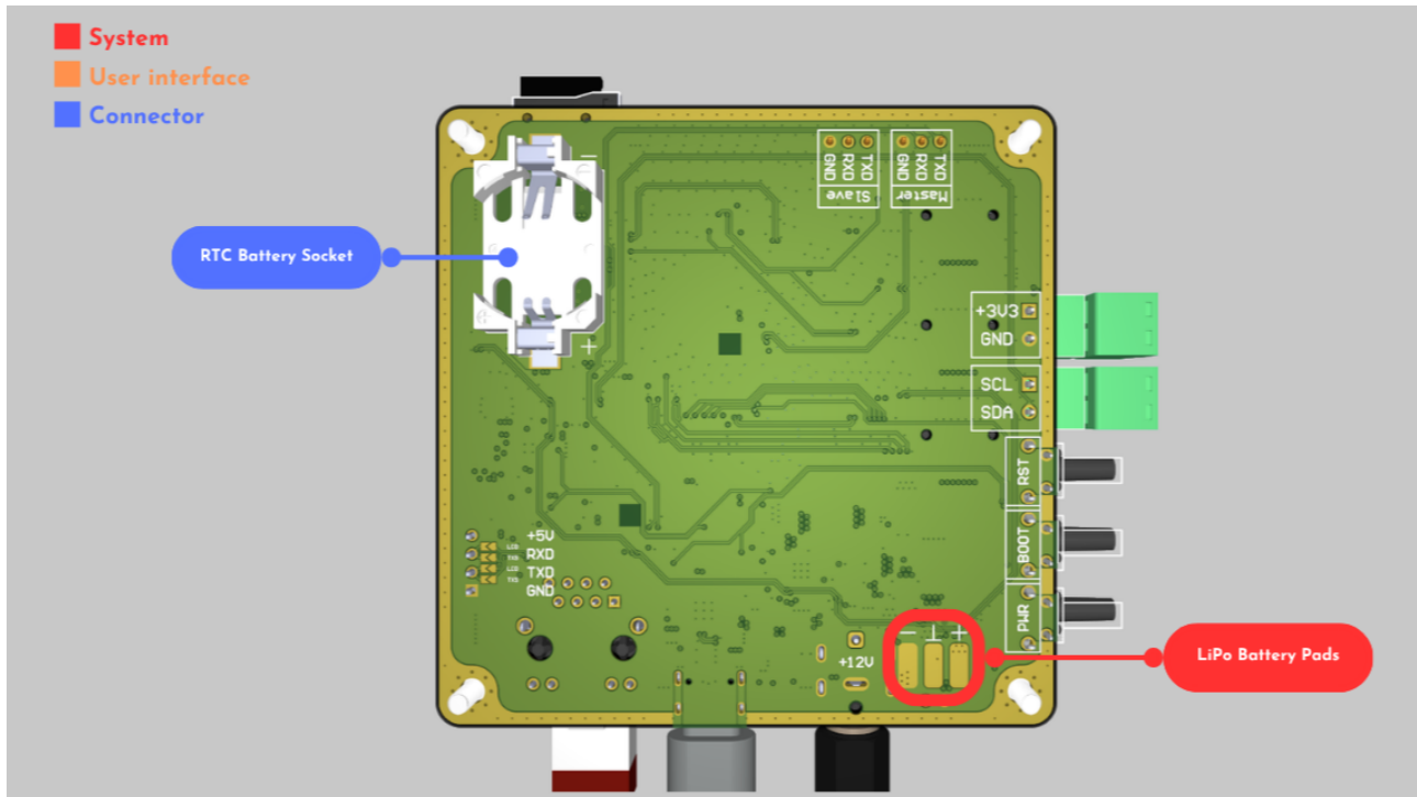
Hình 7.2: Bottom Assembly Diagram
