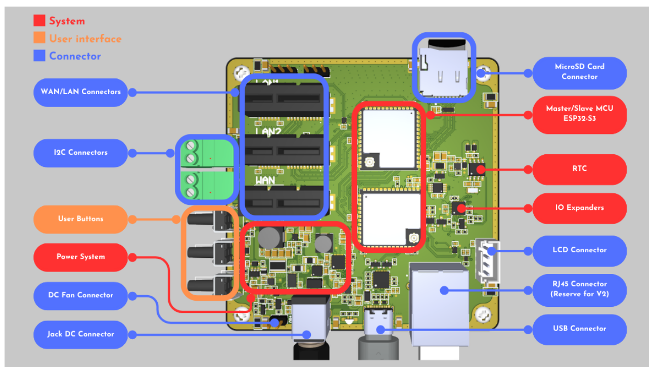
Hình 7.1: Top Assembly Diagram
