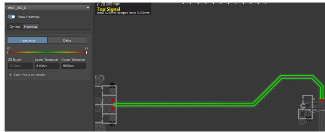
Hình 4.55: Biểu đồ phân bố trở kháng (Impedance Heatmap) đường vi sai.
