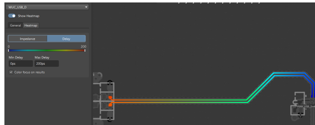
Hình 4.56: Biểu đồ phân bố độ trễ lan truyền (Propagation Delay) đường vi sai.
