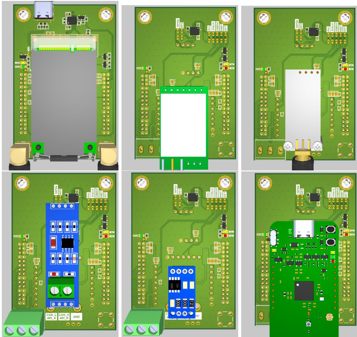
Hình 7.4: Các Module Adapter đang hỗ trợ.
