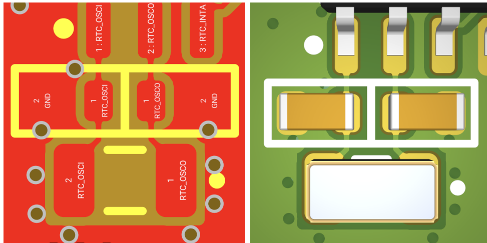
Hình 4.39: Kỹ thuật tạo Guard Ring và via stitching xung quanh khối thạch anh để cô lập nhiễu.
