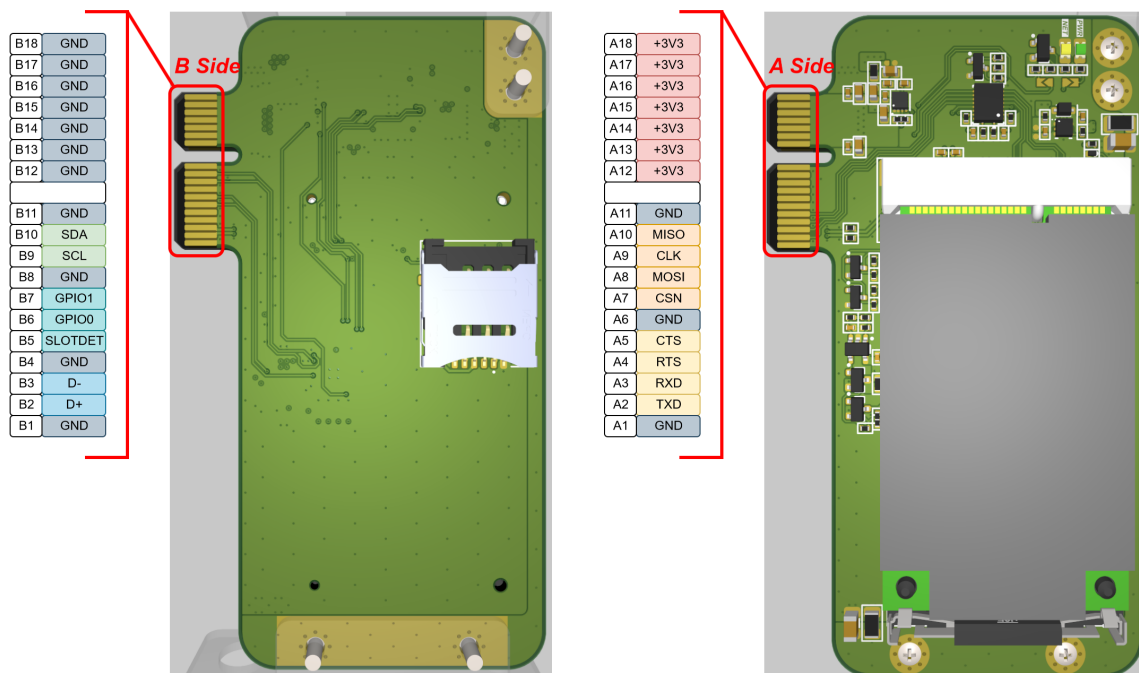
Hình 4.2: Sơ đồ chân Module Adapter
