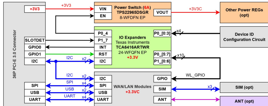
Hình 4.9: Sơ đồ khối mạch adapter
