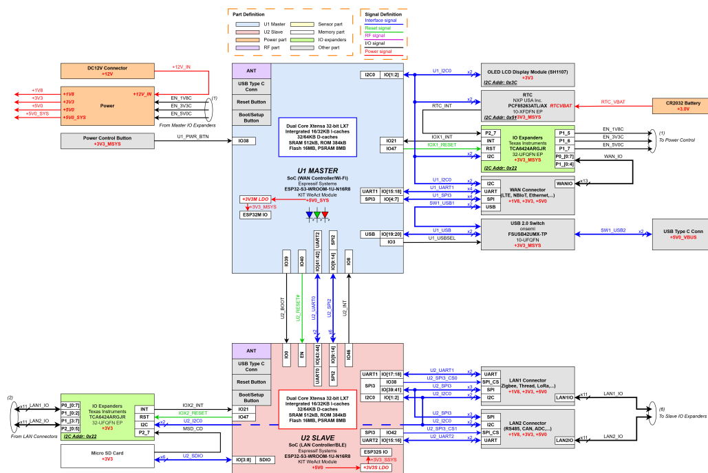
Hình 4.2: Sơ đồ khối Phần cứng
