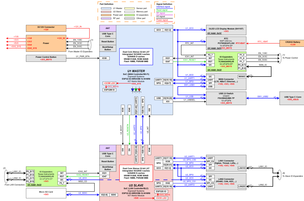
Hình 4.3: Sơ đồ khối Phần cứng
