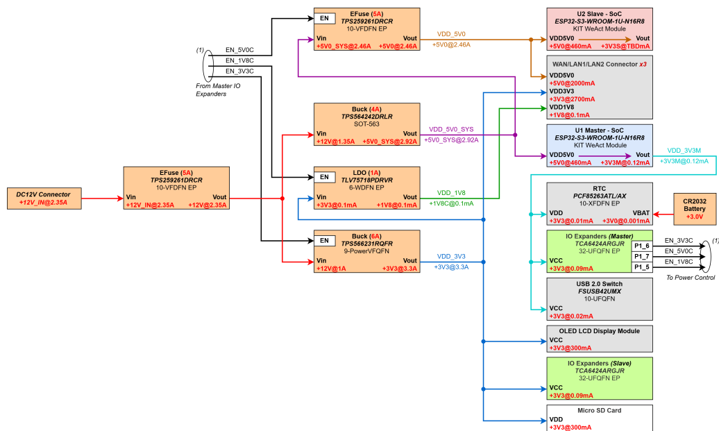
Hình 4.4: Sơ đồ hệ thống nguồn
